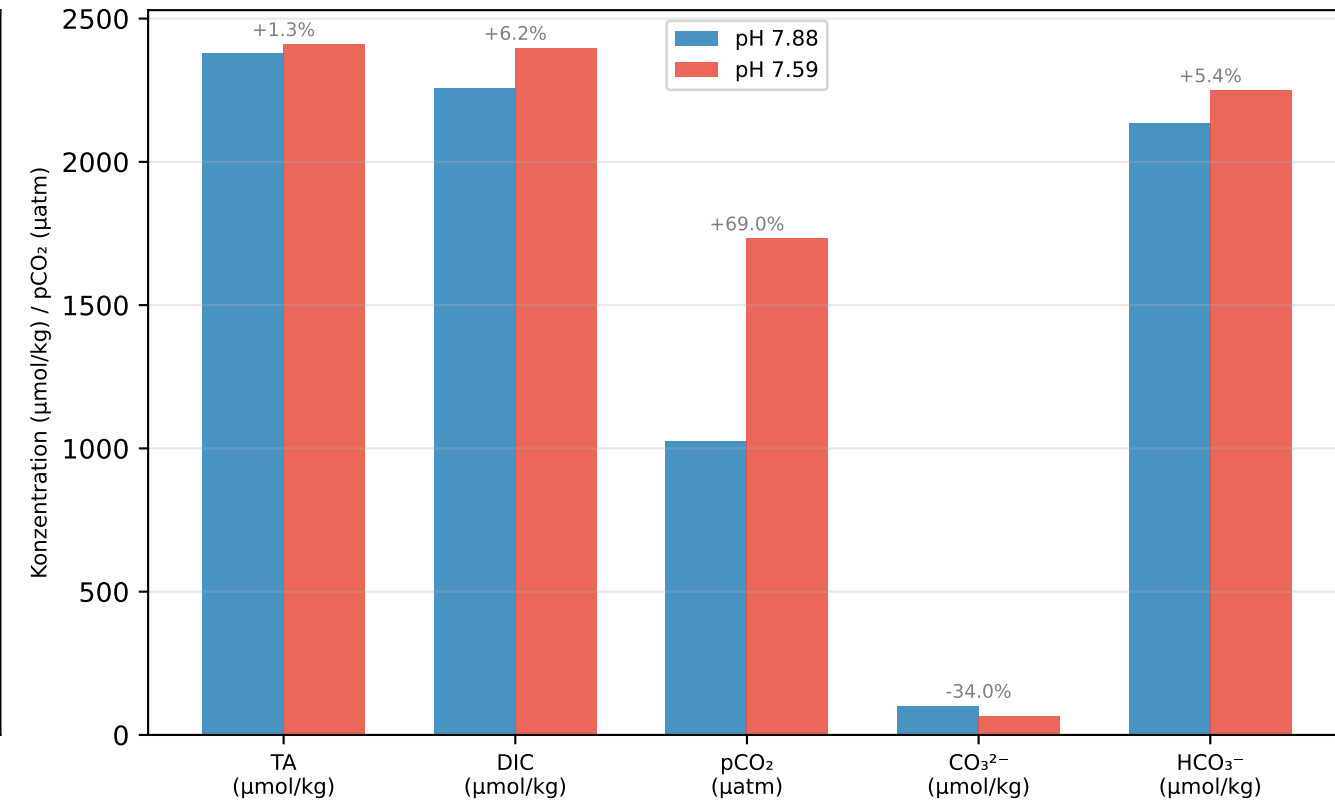
D) Karbonat-Systemparameter bei beiden Versauerungsszenarien (CO 2 SYS v3.0)
