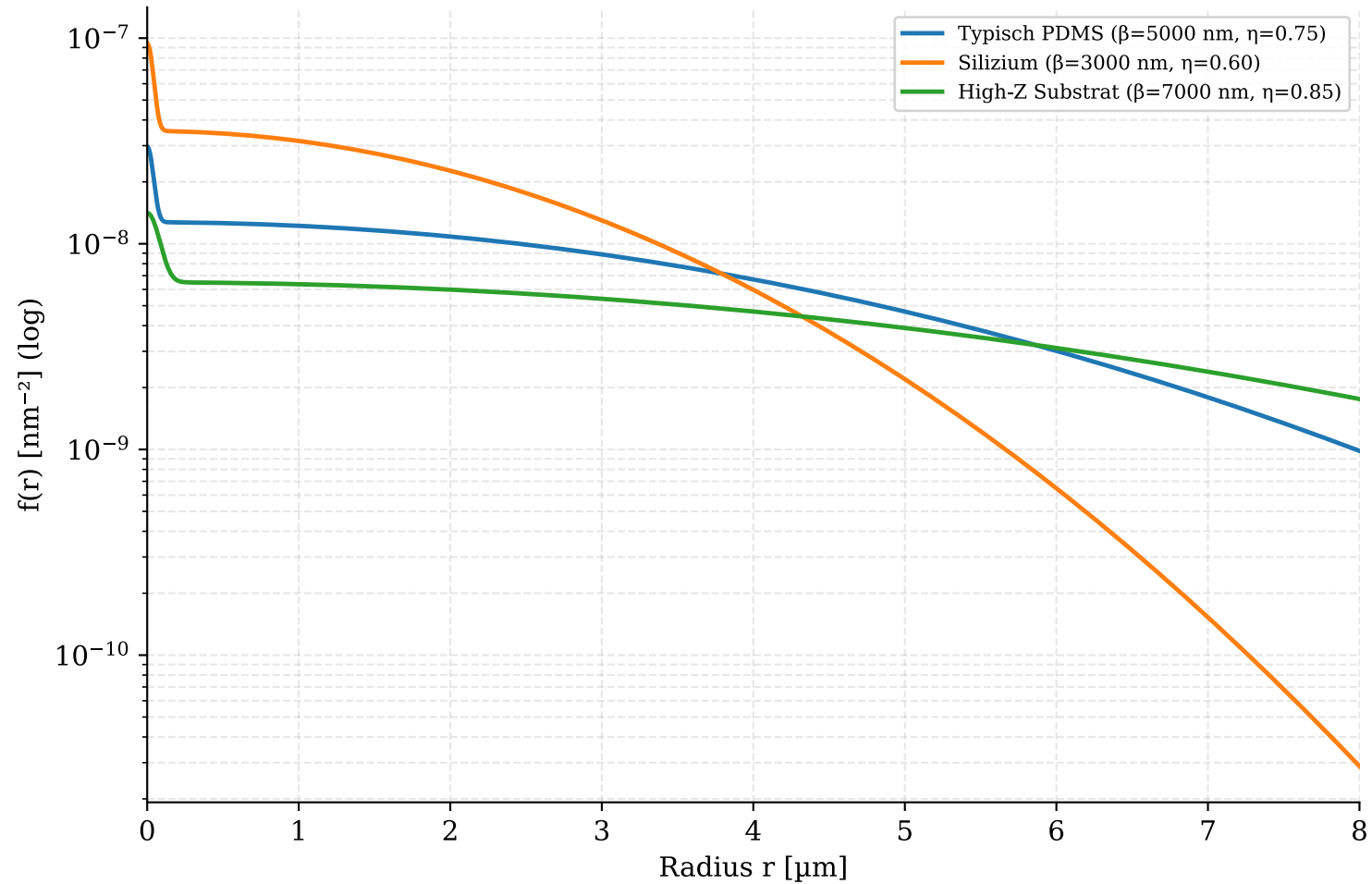
Proximitätsfunktion f(r) : Vorwärts- und Rückstreuung
