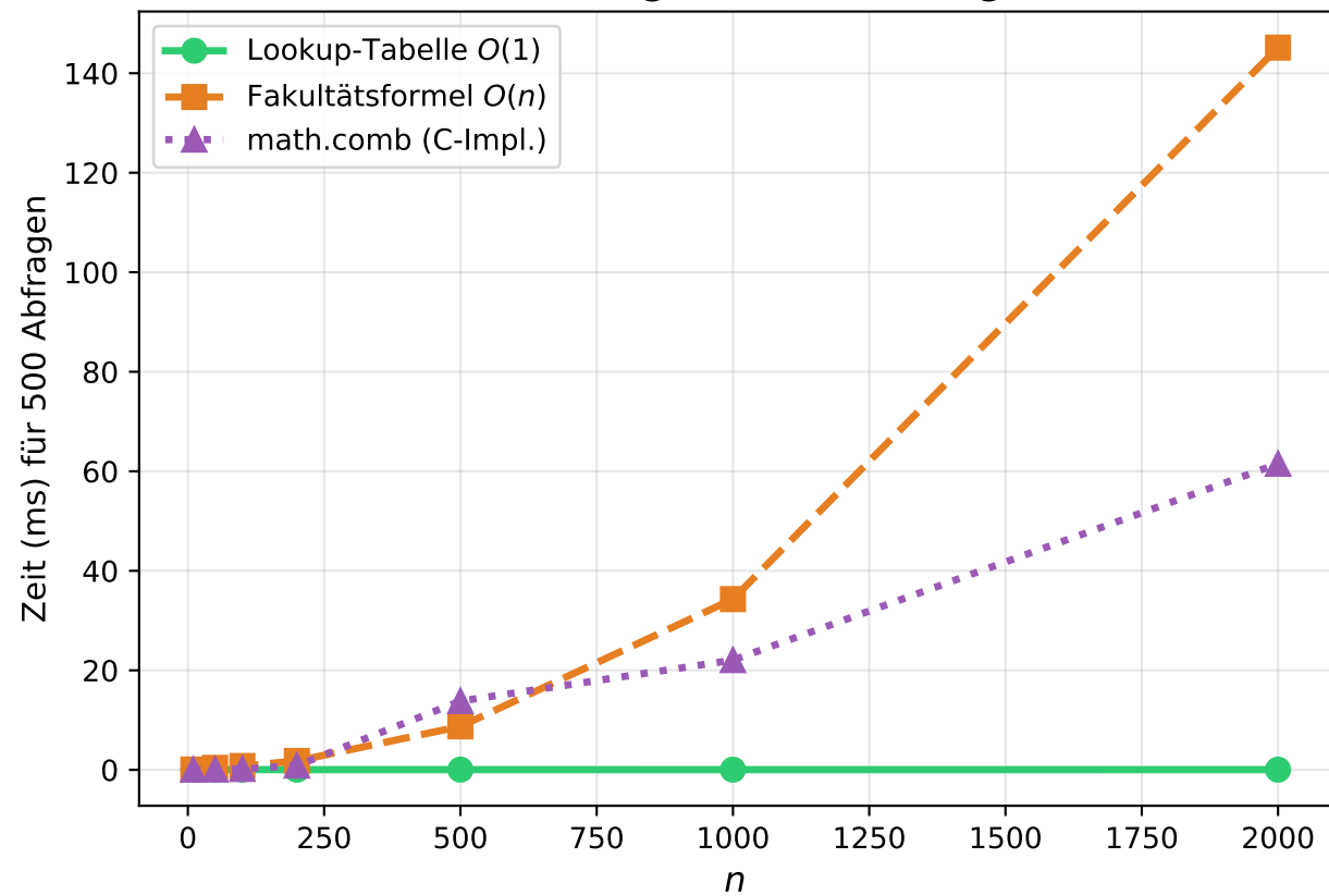
Laufzeitvergleich: 500 Abfragen
