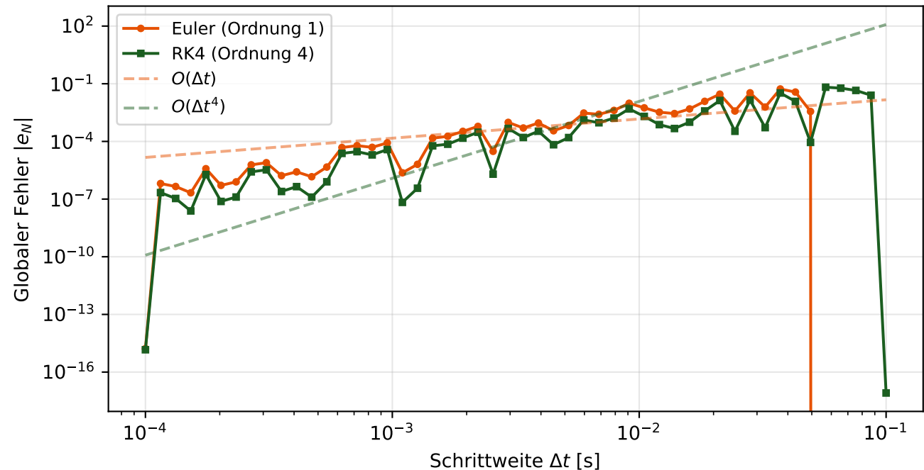
Konvergenzordnung: Euler vs. RK4
