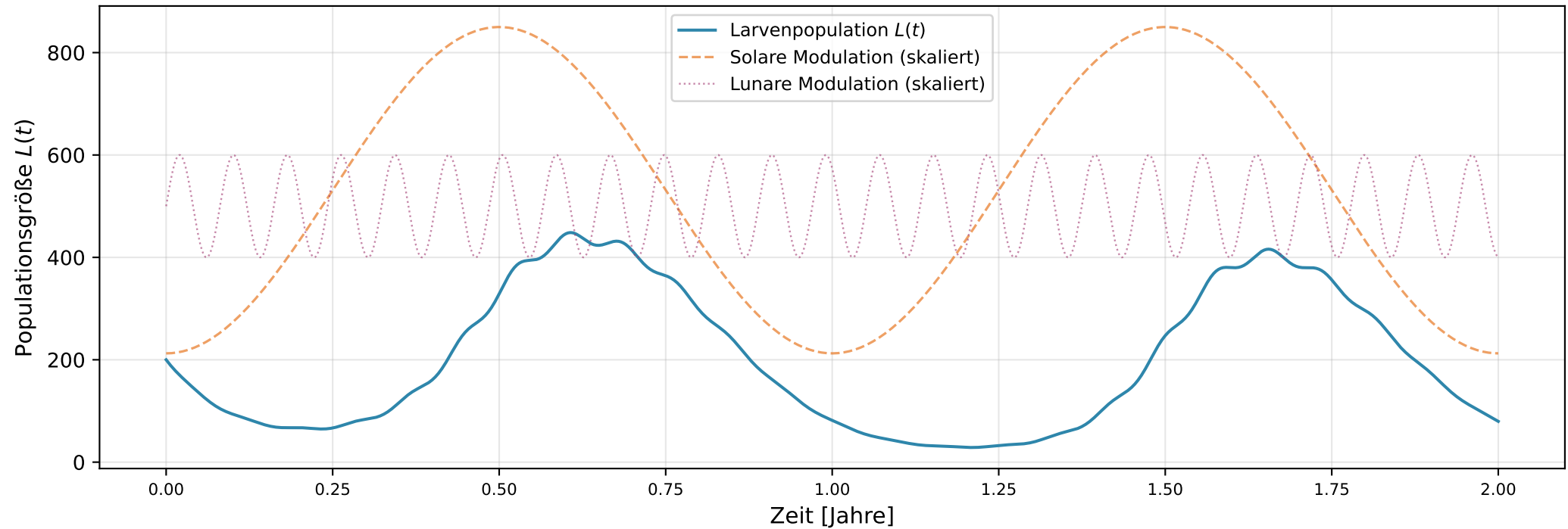
(a) Larvenpopulation mit solarer und lunarer Periodizitätskoppelung
