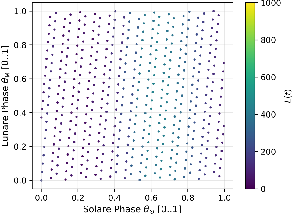
(c) Torus-Projektion: Sonne-Mond-Population
