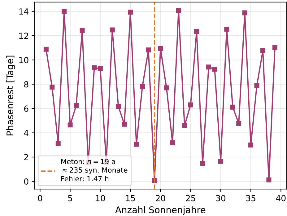
(b) Metonischer Zyklus: 19 Jahre
