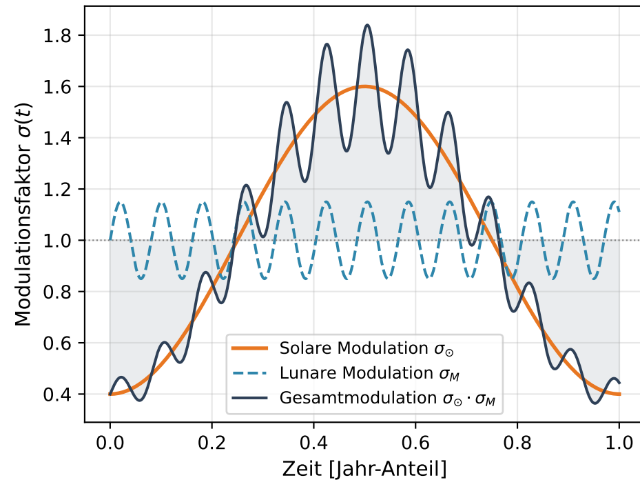
(d) Überlagerte Modulation (Sonne + Mond)
