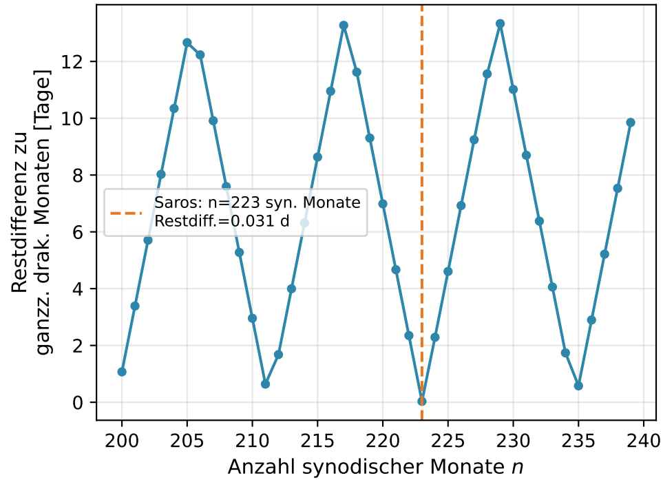
(a) Saros-Zyklus: Kommensurabilität
