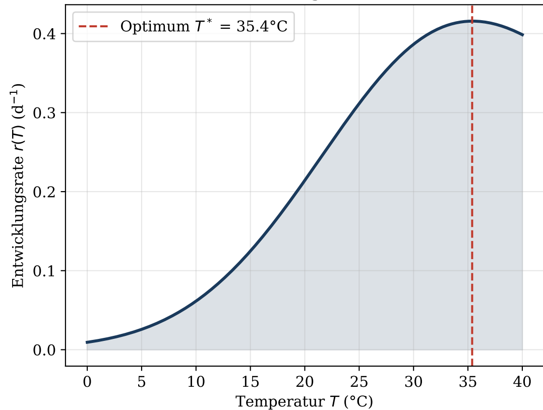
Abb. 4a - Sharpe-Schoolfield: Temperaturabhängige Entwicklungsrates r(T)
