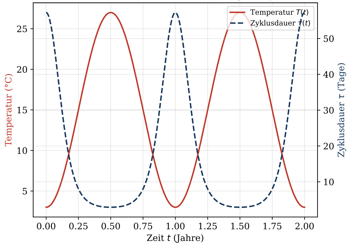
Abb. 4b - Saisonale Modulation und Zyklusperiode \tau(t)
