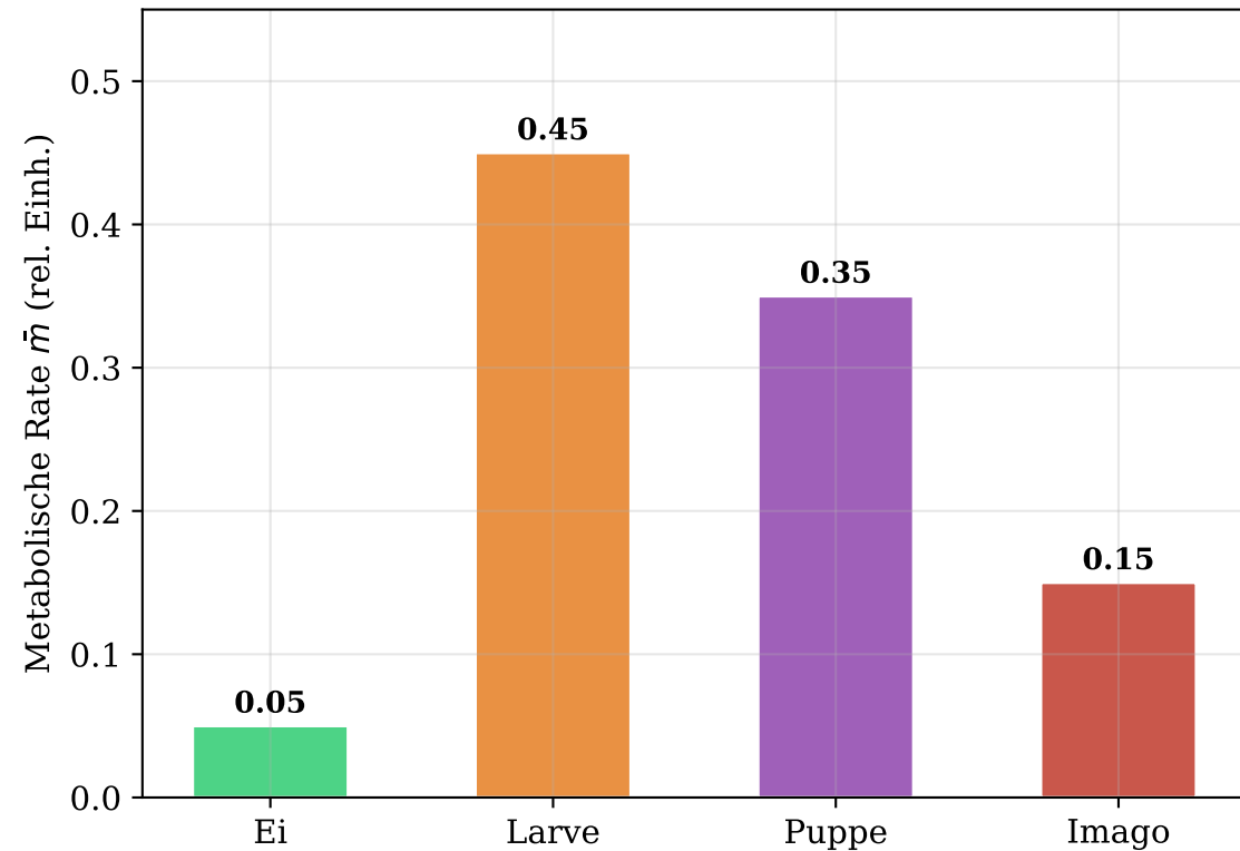
Abb. 6b - Mittlere metabolische Rate \bar{m} pro Metamorphosephase
