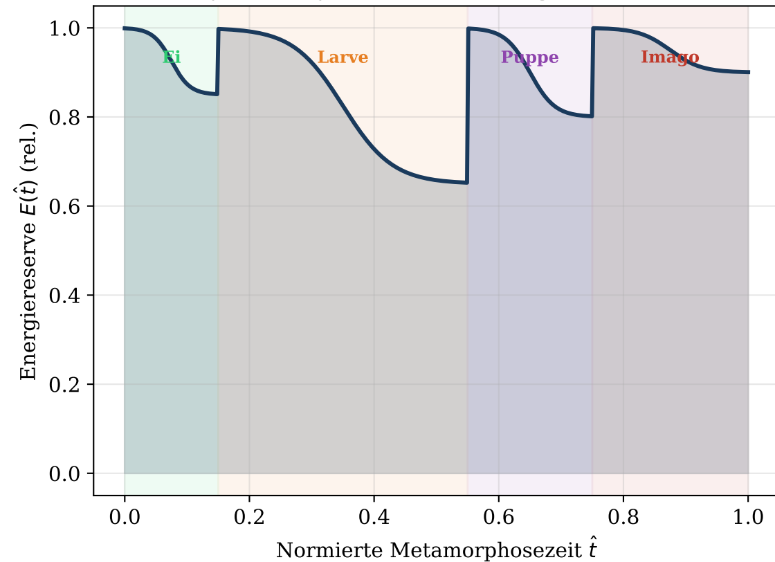
Abb. 6a - Energiereserven E(t) im holometabolen Zyklus (dynamisches Budgetmodell)
