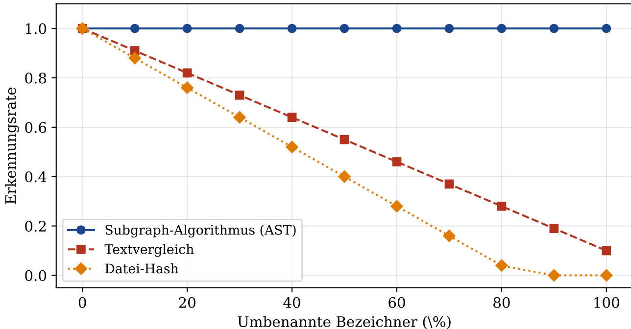
Plagiatserkennungsrate nach Variablenumbenennung
