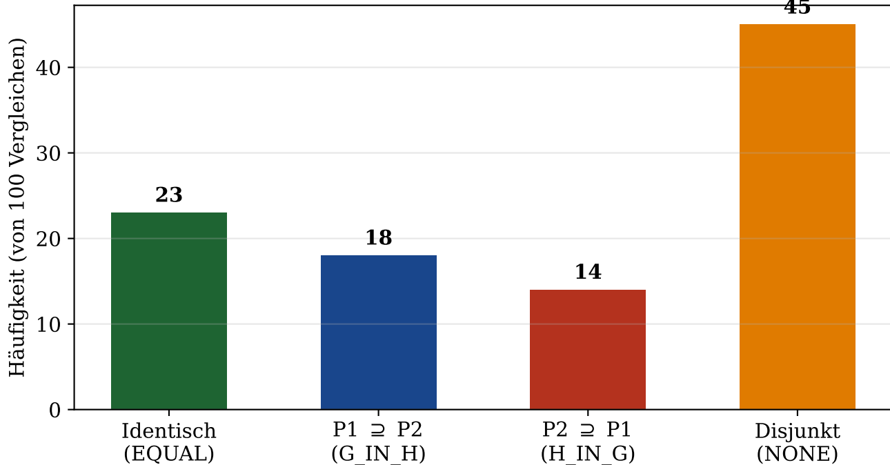
Verteilung der Subgraph-Verifikationsergebnisse
