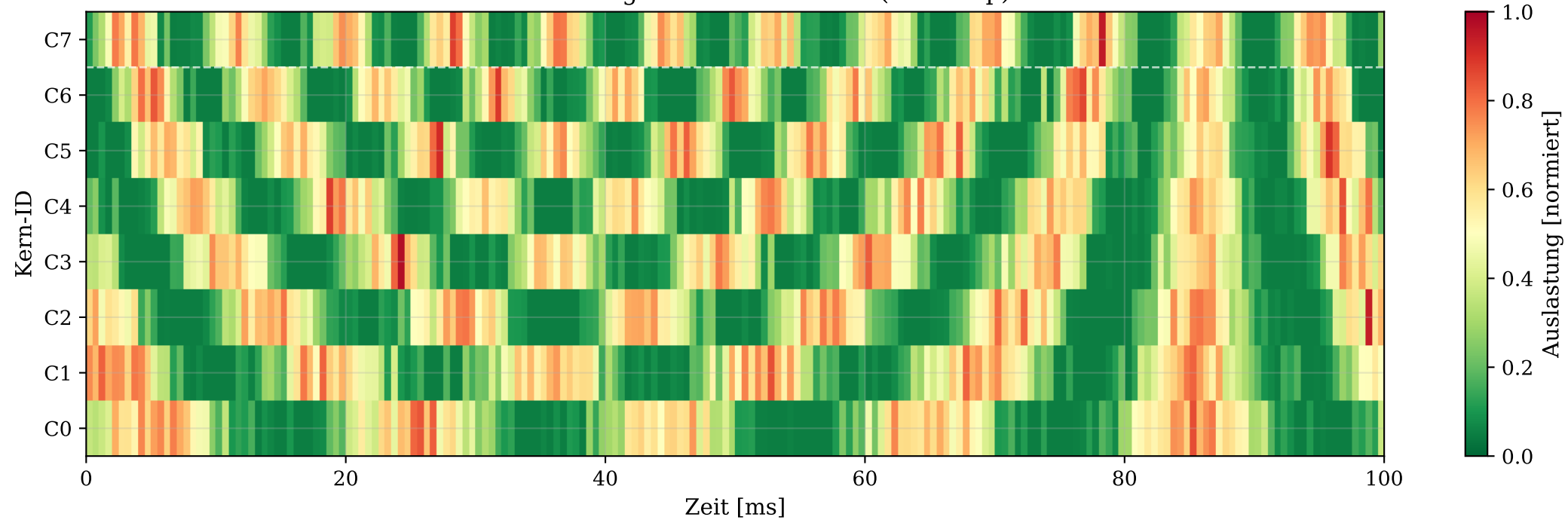
Lastverteilung ueber alle 8 Kerne (Heatmap)
