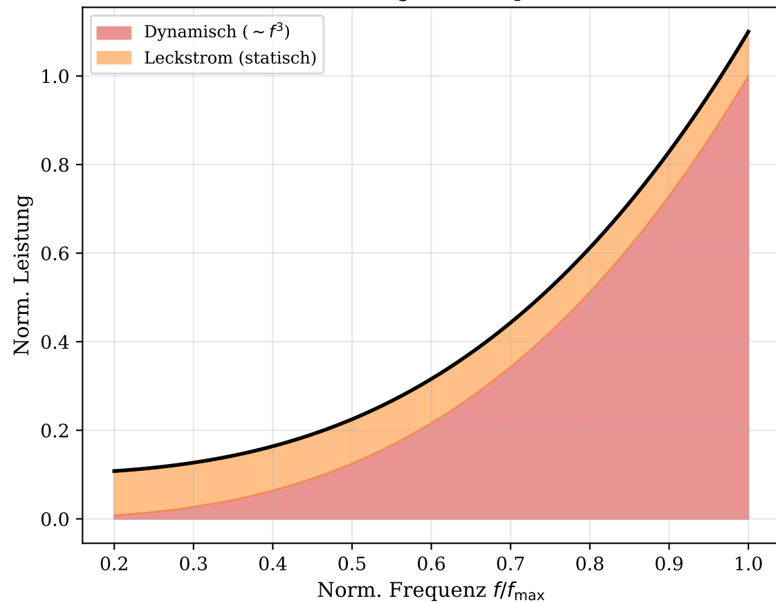
DVFS-Leistungsmodell (pro Kern)
