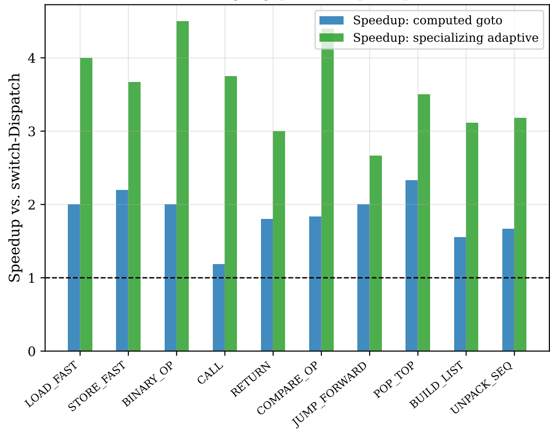
Beschleunigungspotenzial pro Opcode
