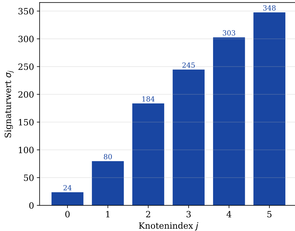
Signatursequenz \sigma^S des Spin-Netzwerks
