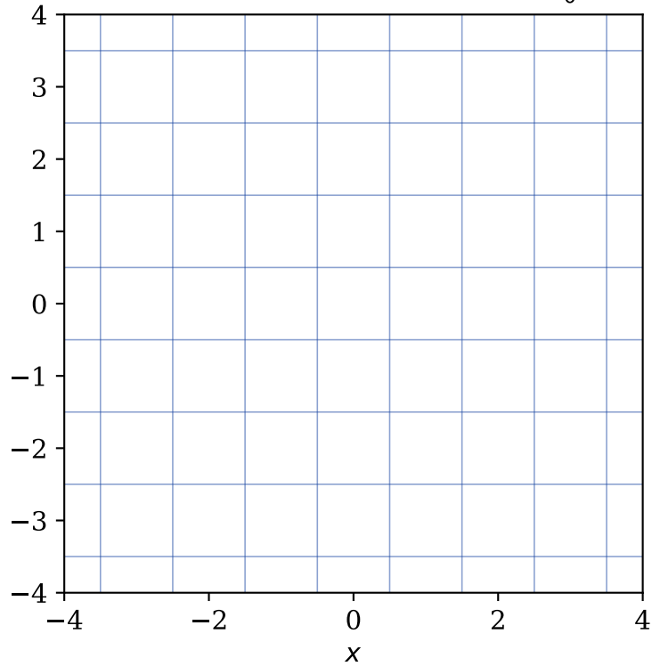
Vor Masse: flache Raumzeit G_0
