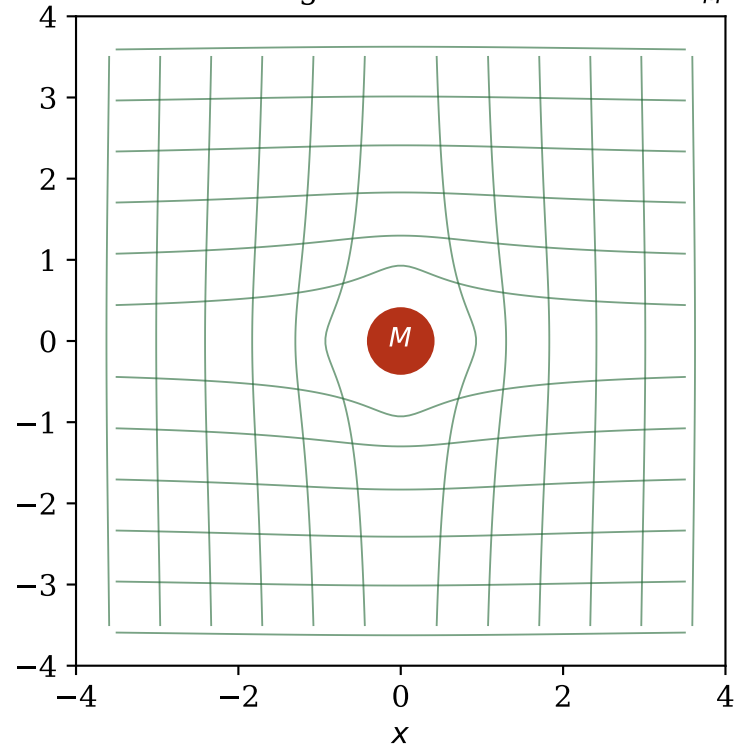
Nach Masse: gekrueemte Raumzeit G_M
