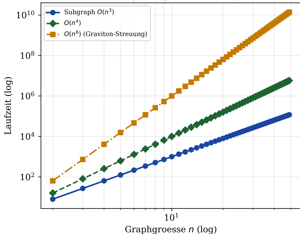
Skalierung fuer grosse QG-Graphen
