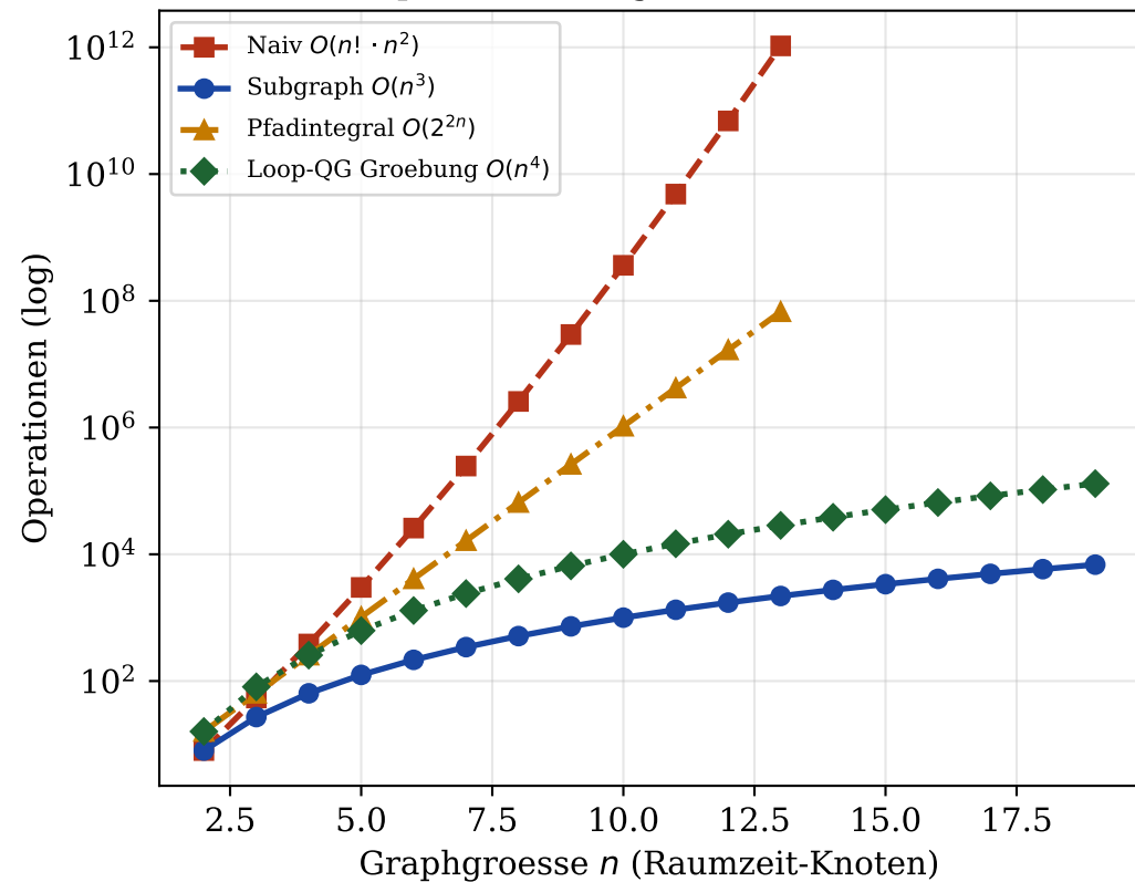
Komplexitaetsvergleich QG-Ansaetze
