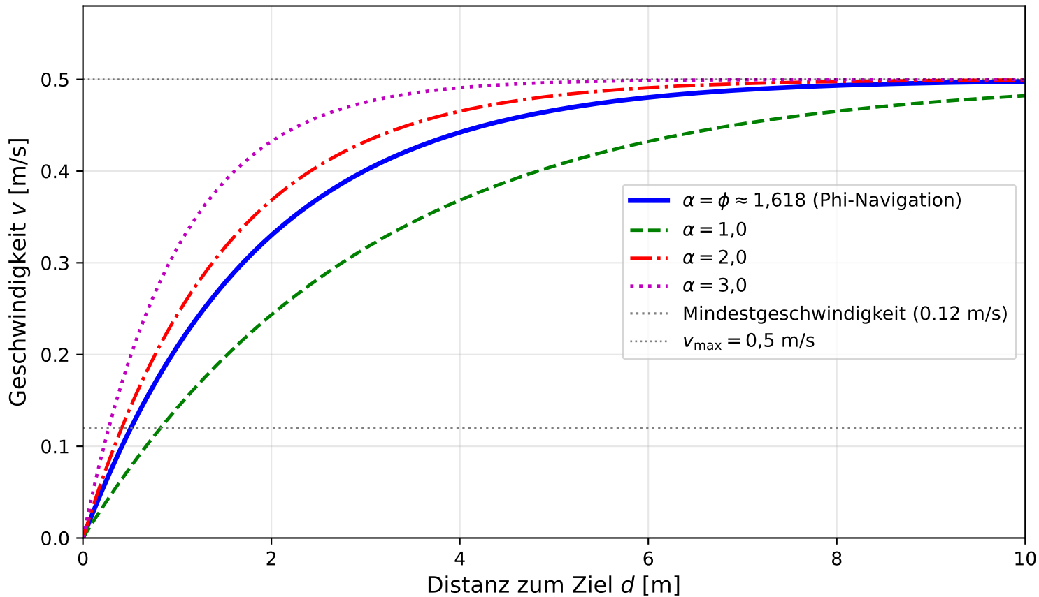
Phi-gewichtetes Geschwindigkeitsprofil ( d_{\text{ref}} = 3,0 m)
