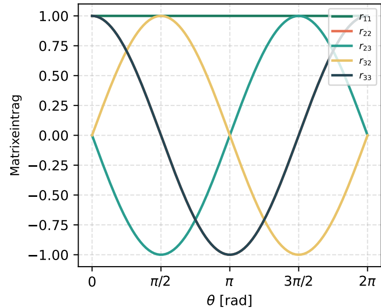
Roll R_x(\theta)
