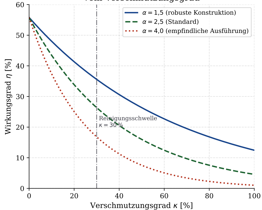
Wirkungsgrad in Abhängigkeit vom Verschmutzungsgrad
