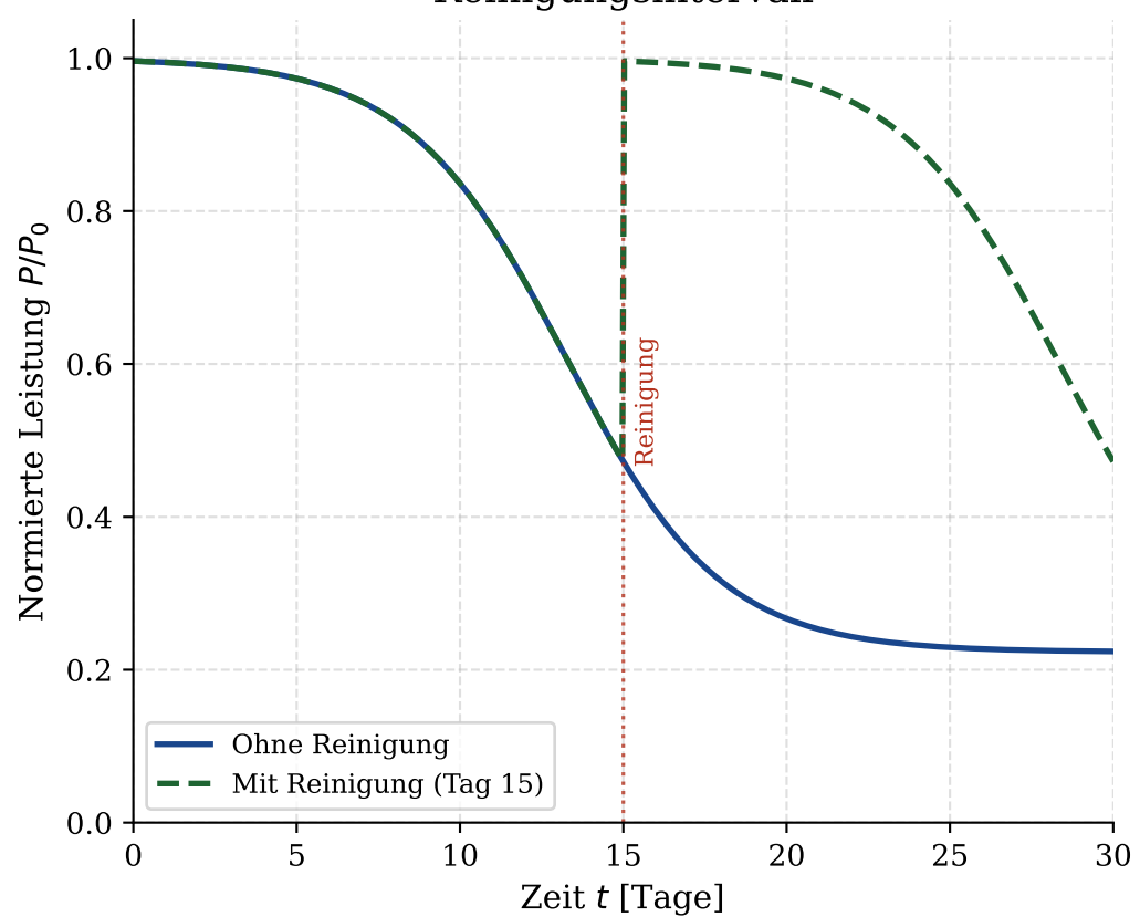
Leistungsverlauf mit und ohne Reinigungsintervall
