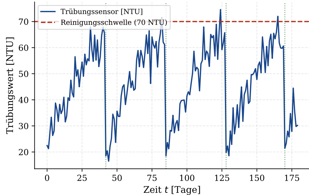
(a) Sensorverlauf: Trübungsgrad
