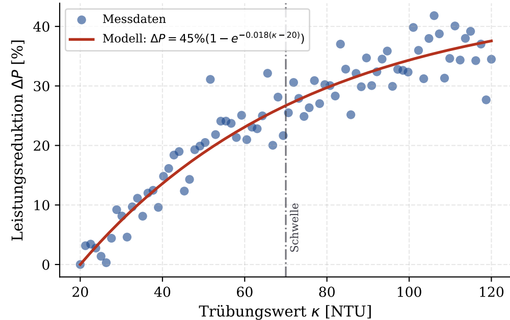
(b) Korrelation: Trübung — Leistungsverlust
