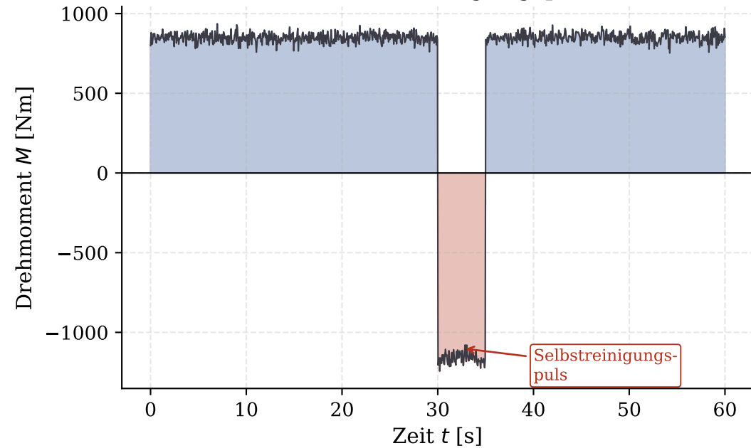
(d) Drehmomentsensor: Normalbetrieb und Selbstreinigungspuls
