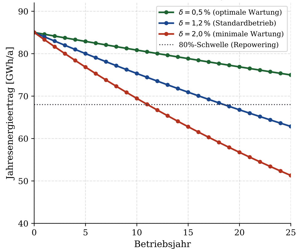
Degradation des Jahresertrags über die Betriebsdauer (25 Jahre)
