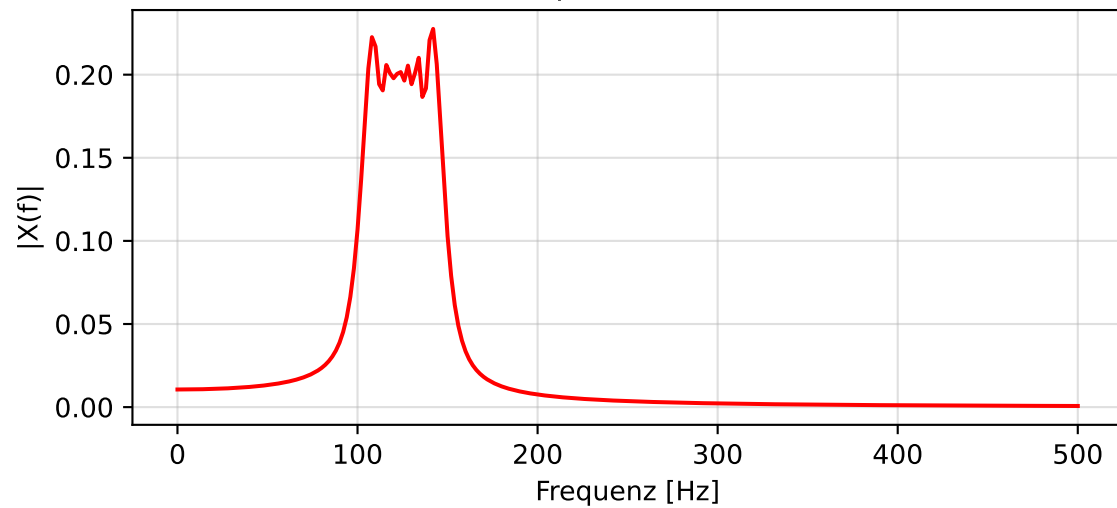
Chirp-Signal (100-150 Hz) (Frequenzbereich)
