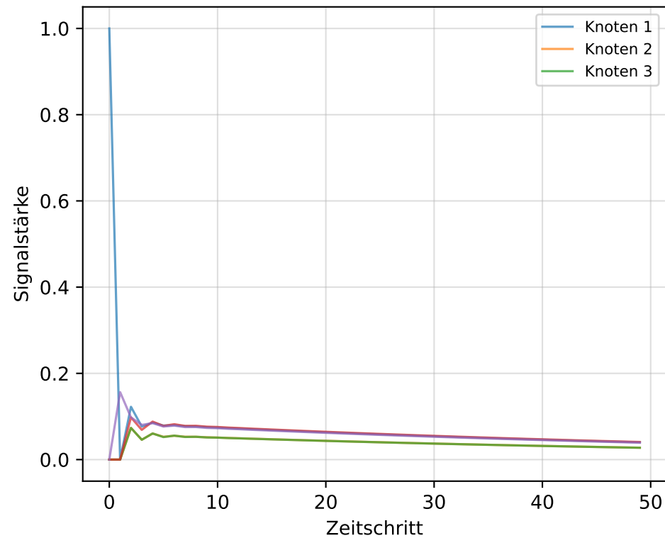
Zufälliges Netzwerk \rho(A) = 0.9844
