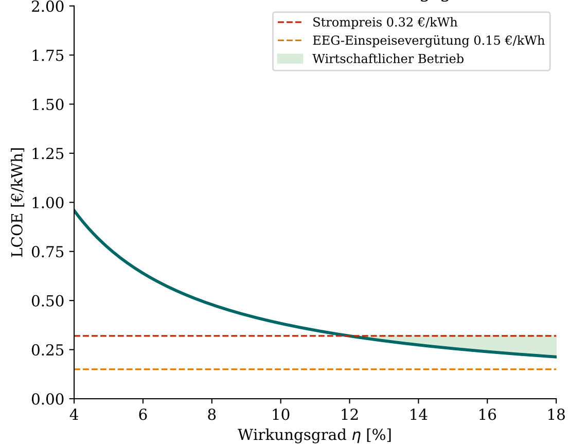
LCOE als Funktion des Wirkungsgrads
