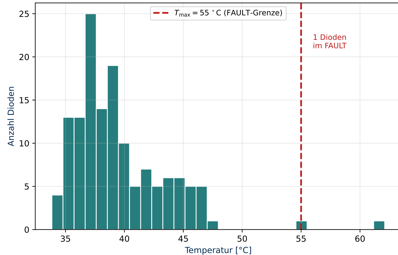
Temperaturhistogramm des Moduls
