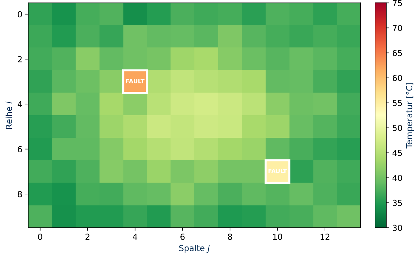
Temperaturverteilung T_{ij} im Dioden-Modul (10 × 14 Dioden, Heatmap)
