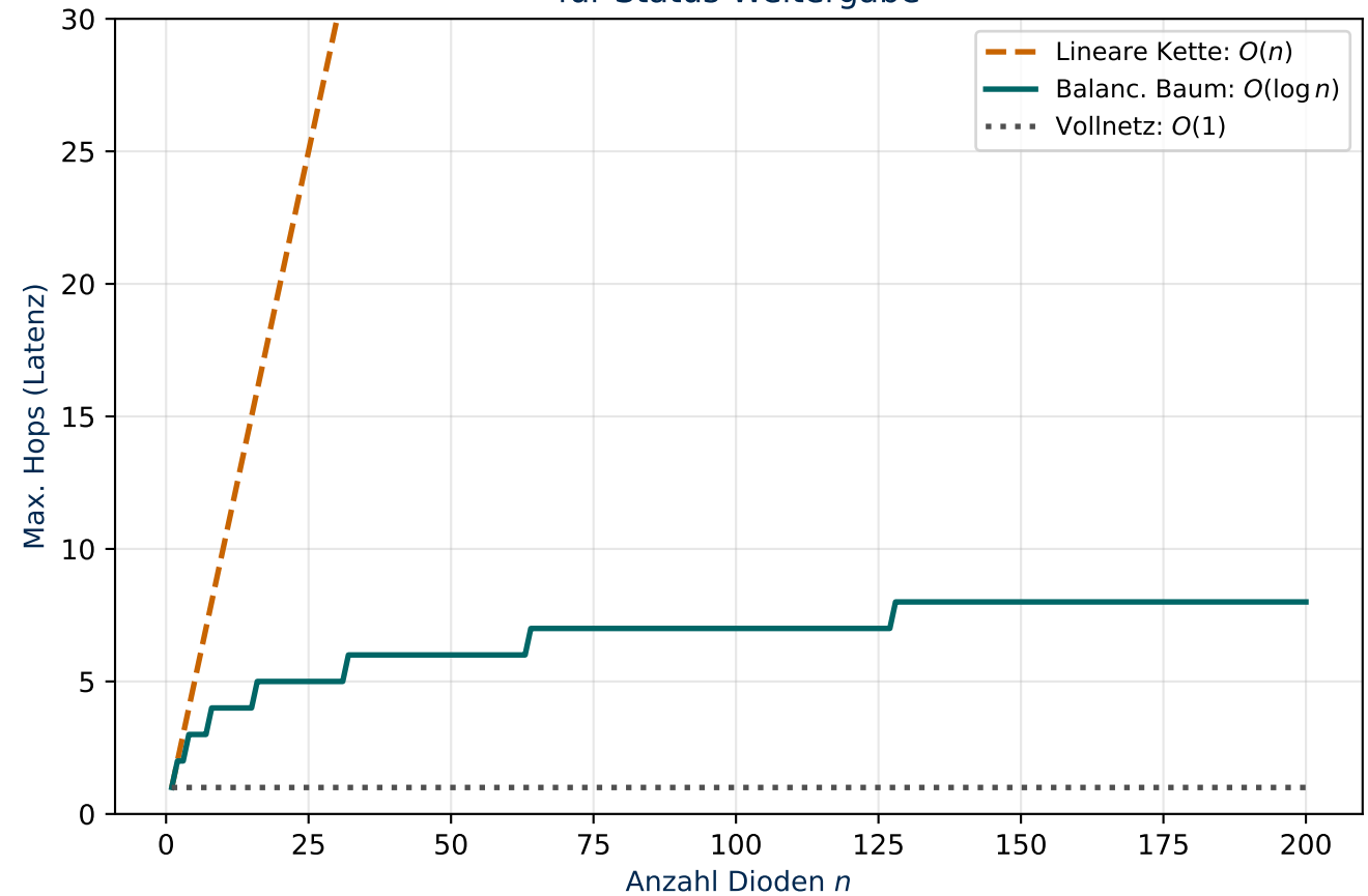
Maximale Routing-Latenz für Status-Weitergabe
