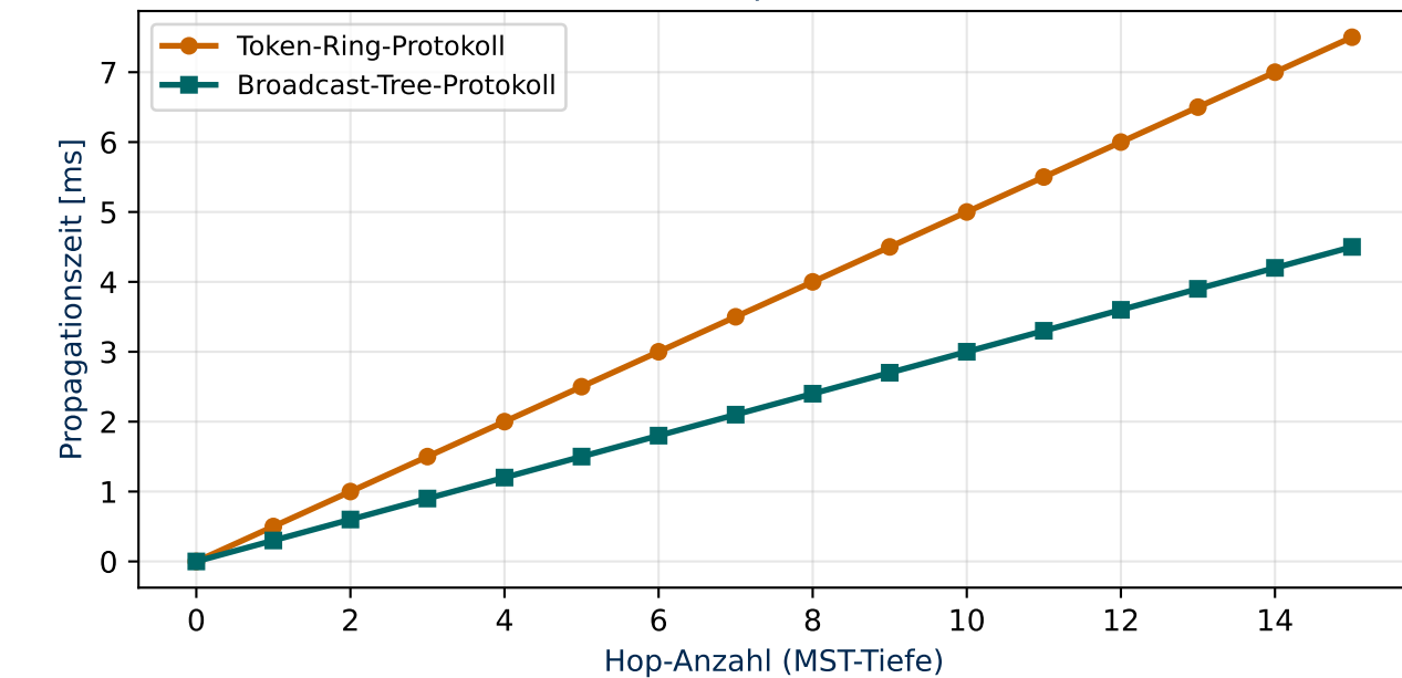
CMD-Propagationszeit vs. Hop-Anzahl
