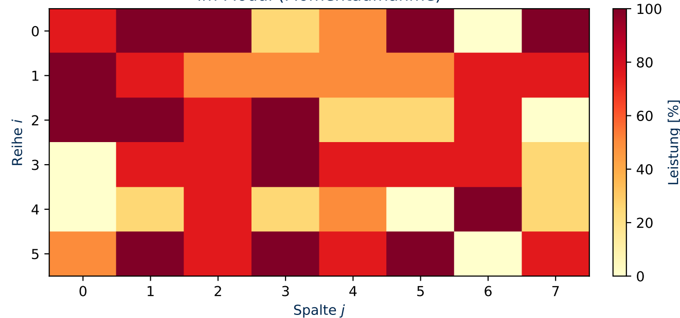
Regelzustand: Leistungsverteilung im Modul (Momentaufnahme)
