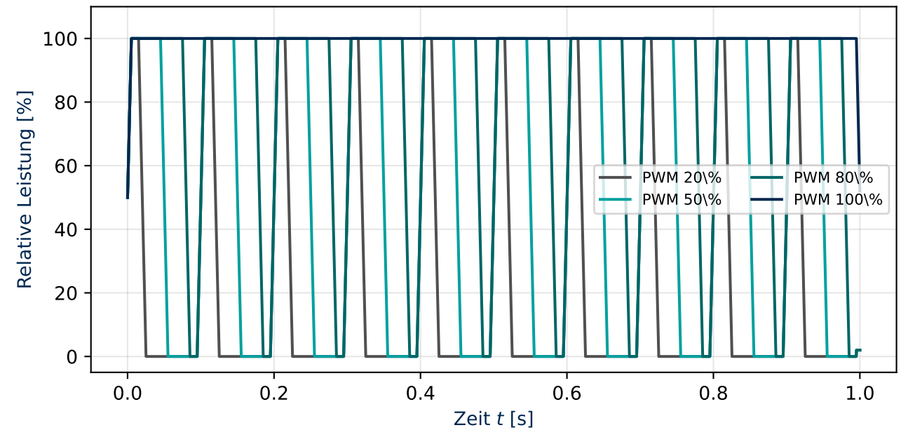
PWM-Dimmung (Schwach / Stark)
