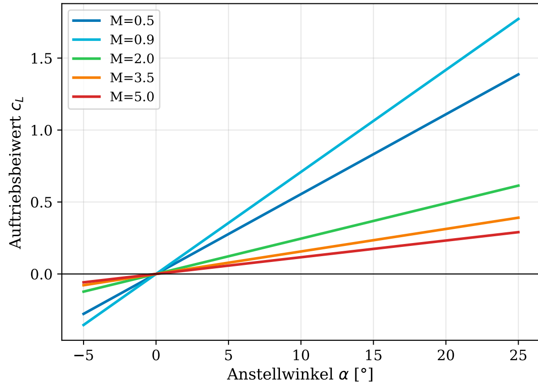
Auftriebscharakteristik
