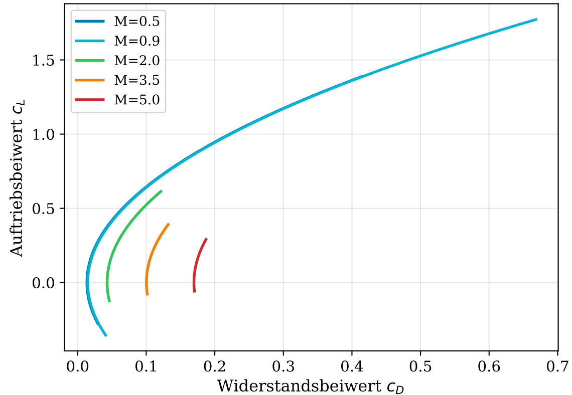
Polare c_L(c_D) — Lilienthal-Polare
