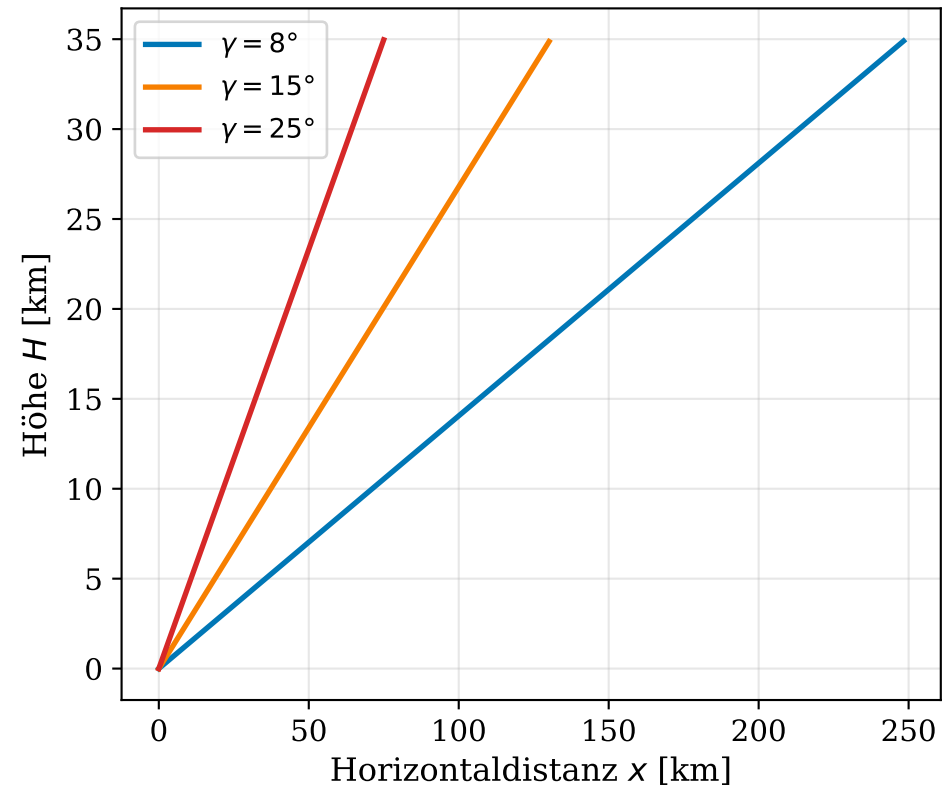
Flugbahn H(x)
