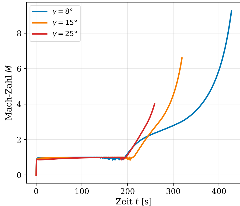
Mach-Verlauf im Steigflug
