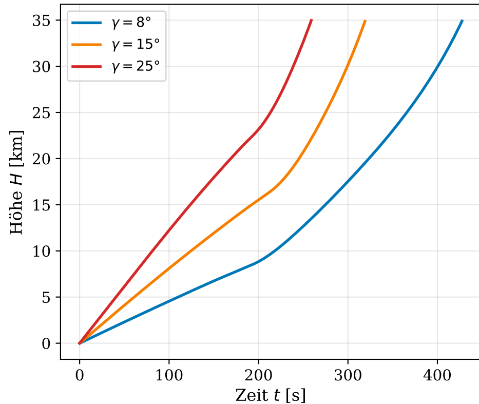
Steigflugprofil H(t)
