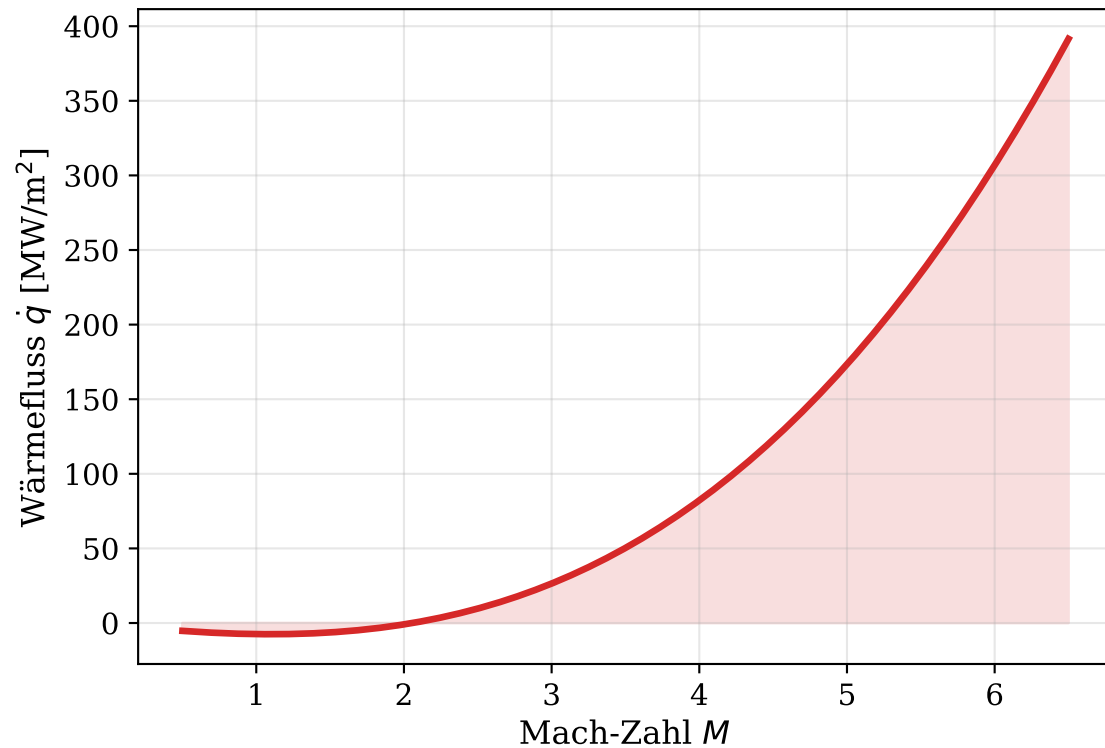
Aerodynamischer Wärmefluss an der Vorderkante ( x_c = 0.5 m)
