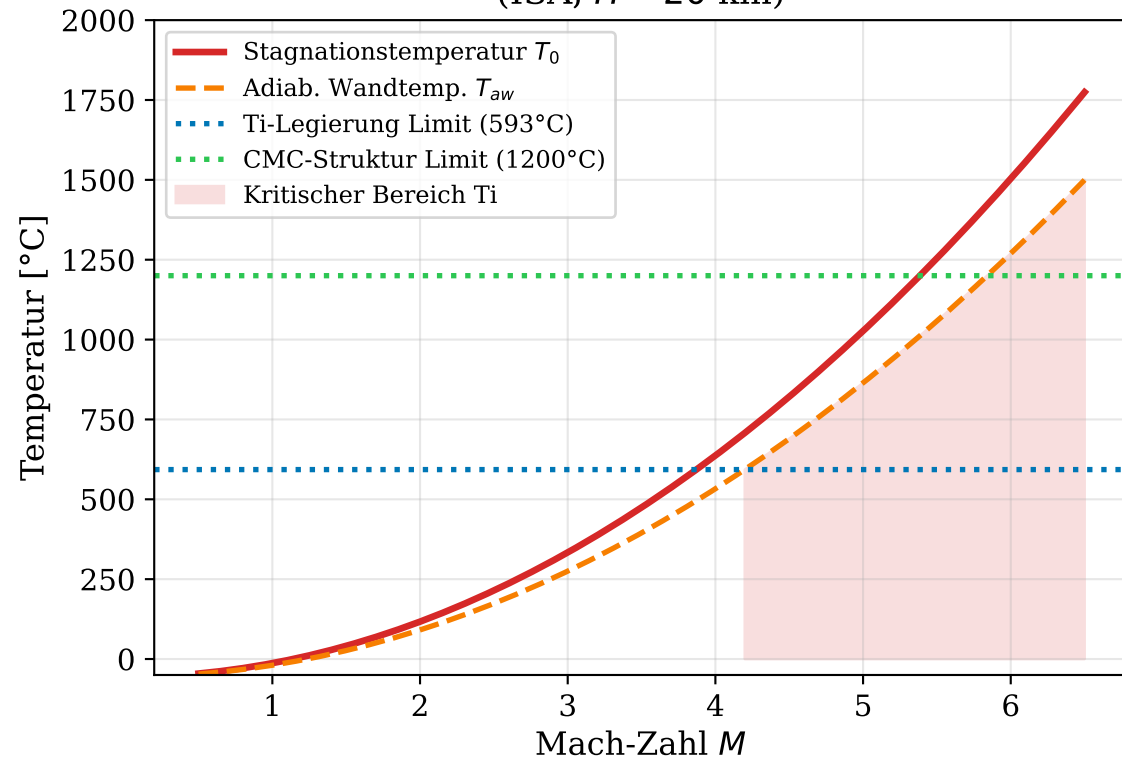
Aerodynamische Erwärmung (ISA, H = 20 km)
