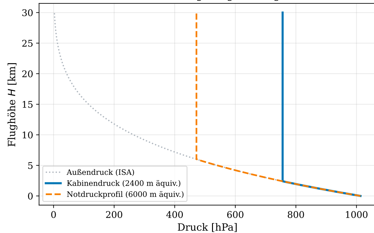
Kabinendruckregelung vs. Flughöhe
