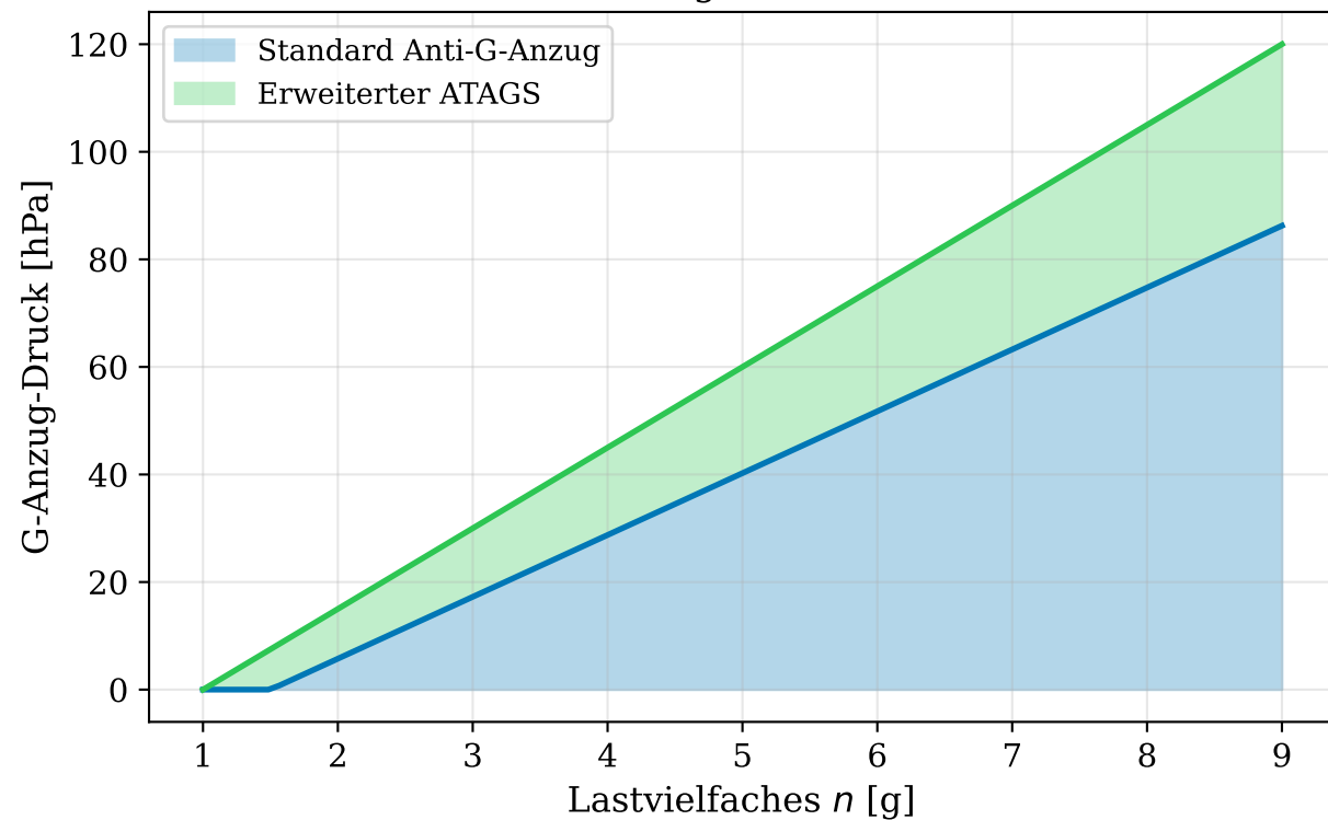
Anti-G-Anzug Druckkennlinie
