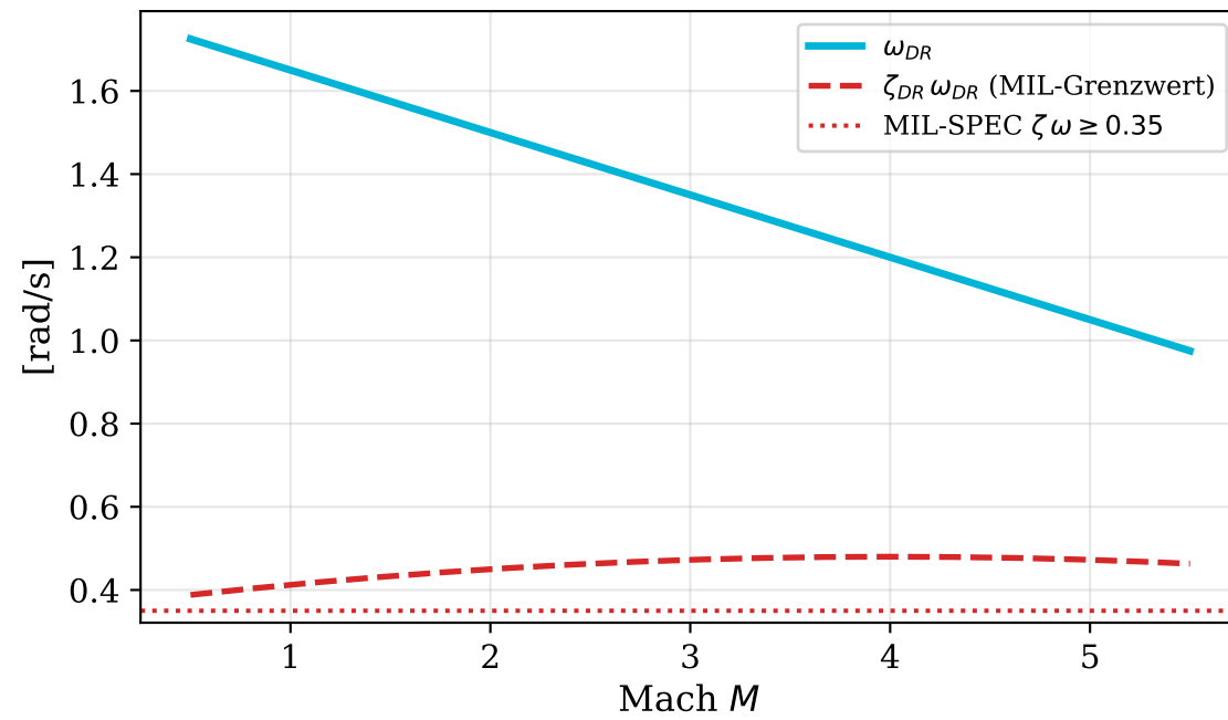
Dutch-Roll Stabilität
