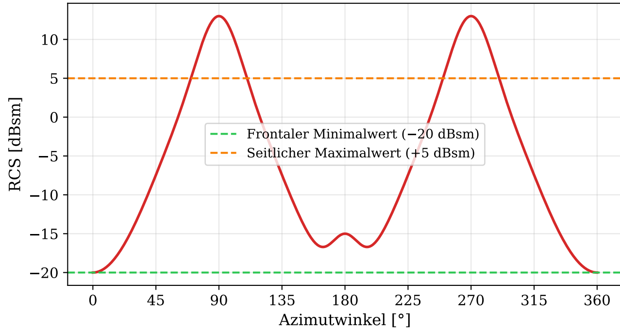
Radar-Querschnitt RCS( \theta )
