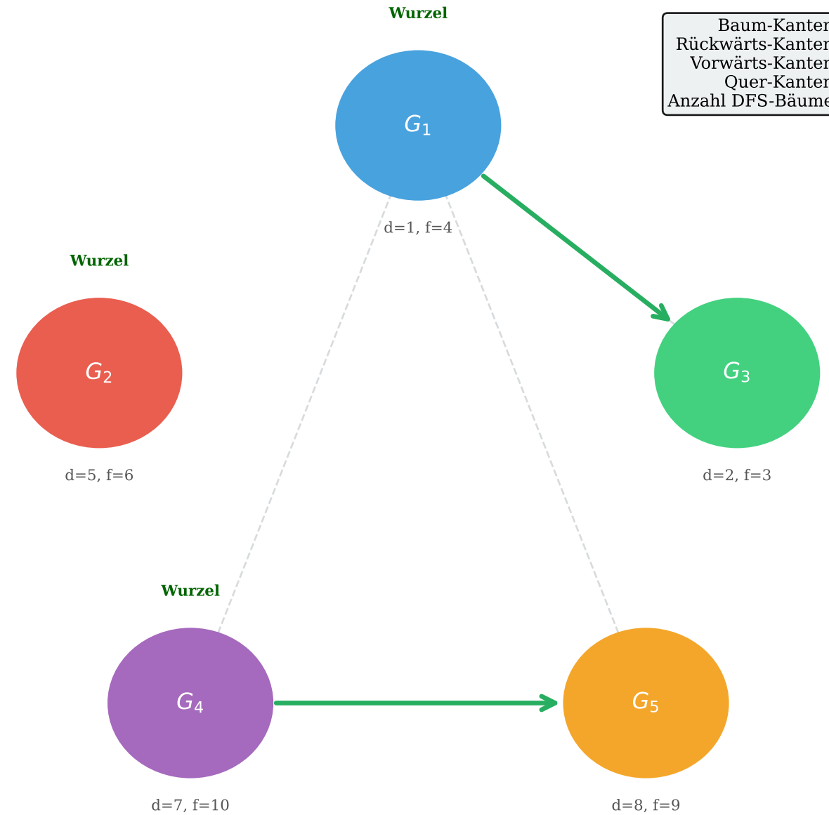
DFS-Wald (Tiefensuche-Bäume)
