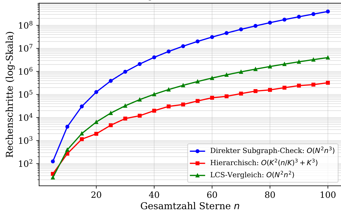
Komplexität vs. Sternanzahl
