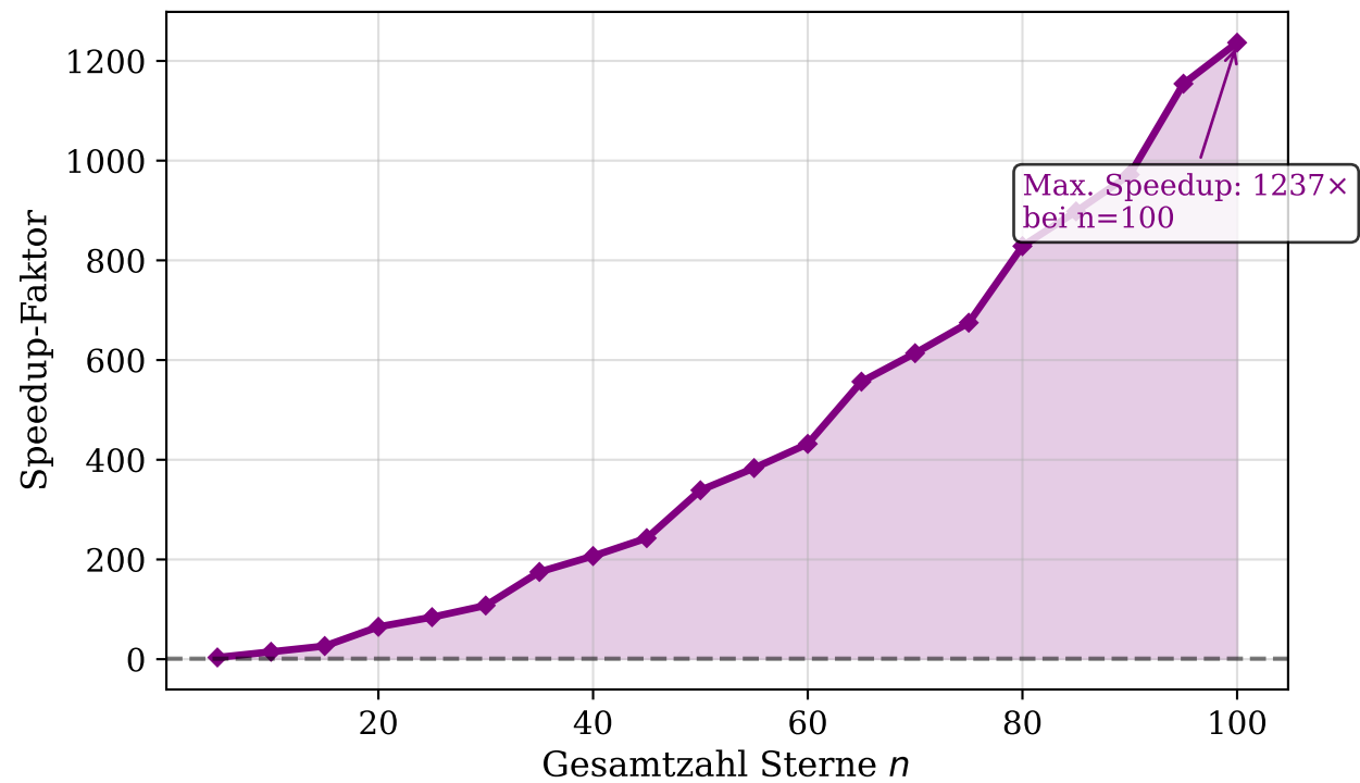
Hierarchischer Speedup-Faktor (Direkt / Hierarchisch)
