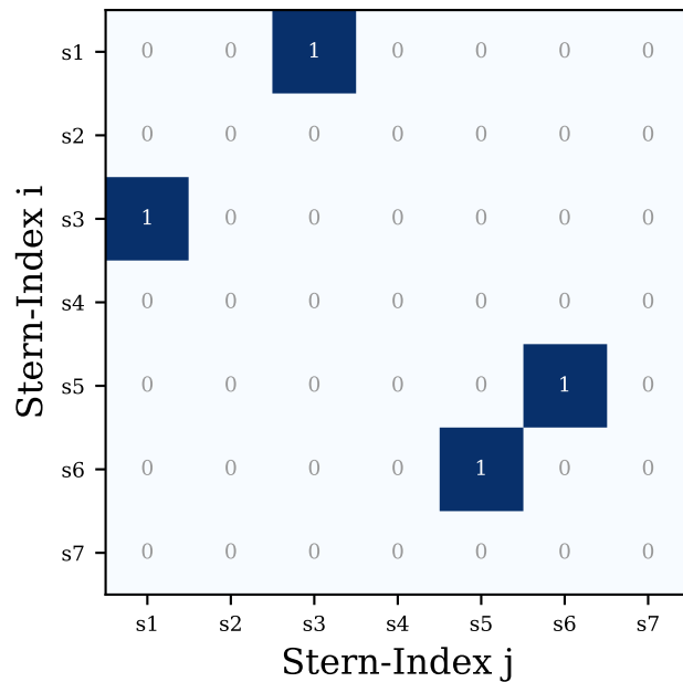
Cluster B (Kugelhaufen)
