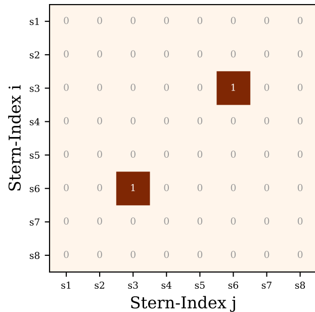
Cluster A (Offener Haufen)
