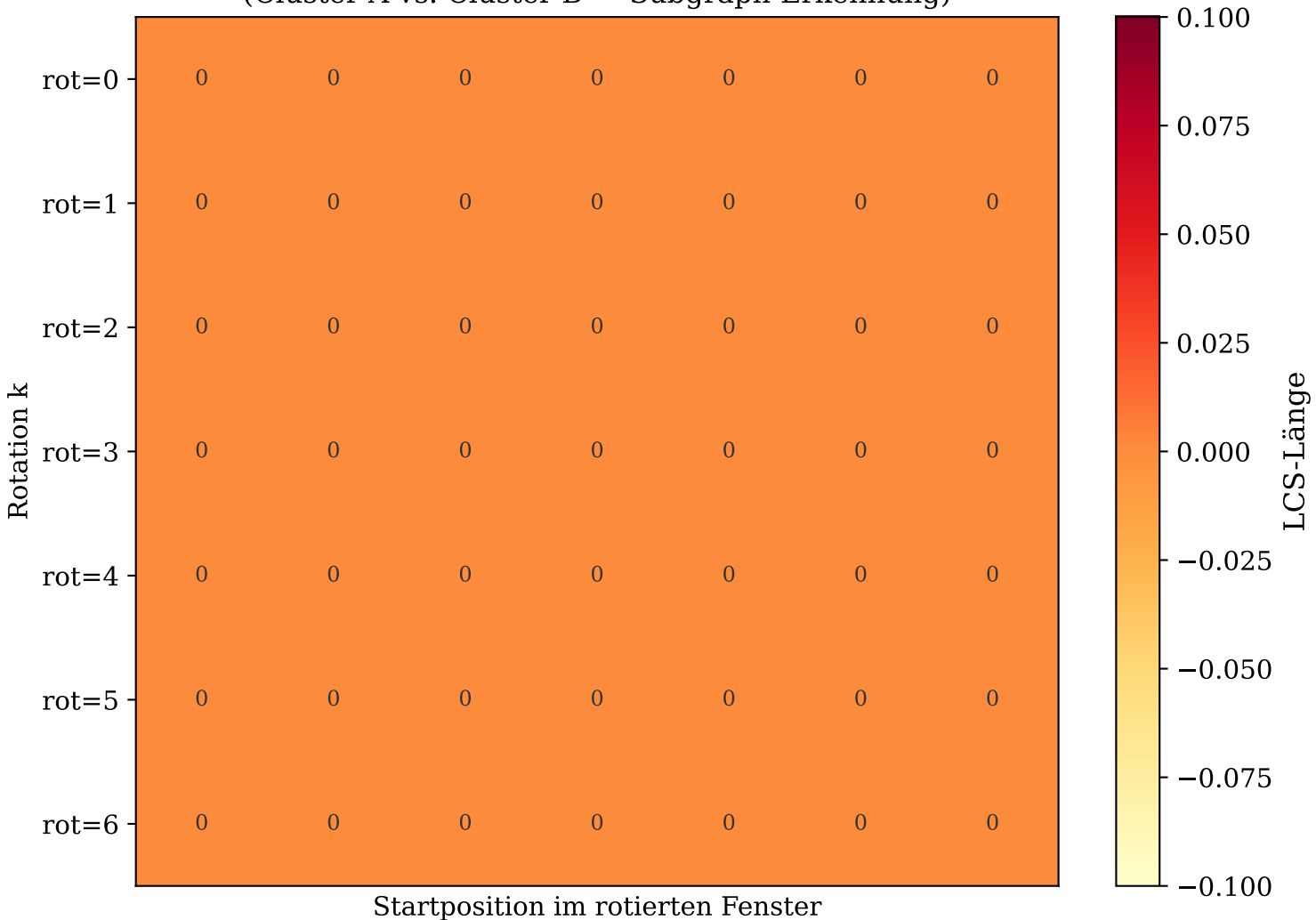
Abbildung 4: LCS-Längen bei allen Rotationen (Cluster A vs. Cluster B — Subgraph-Erkennung)
