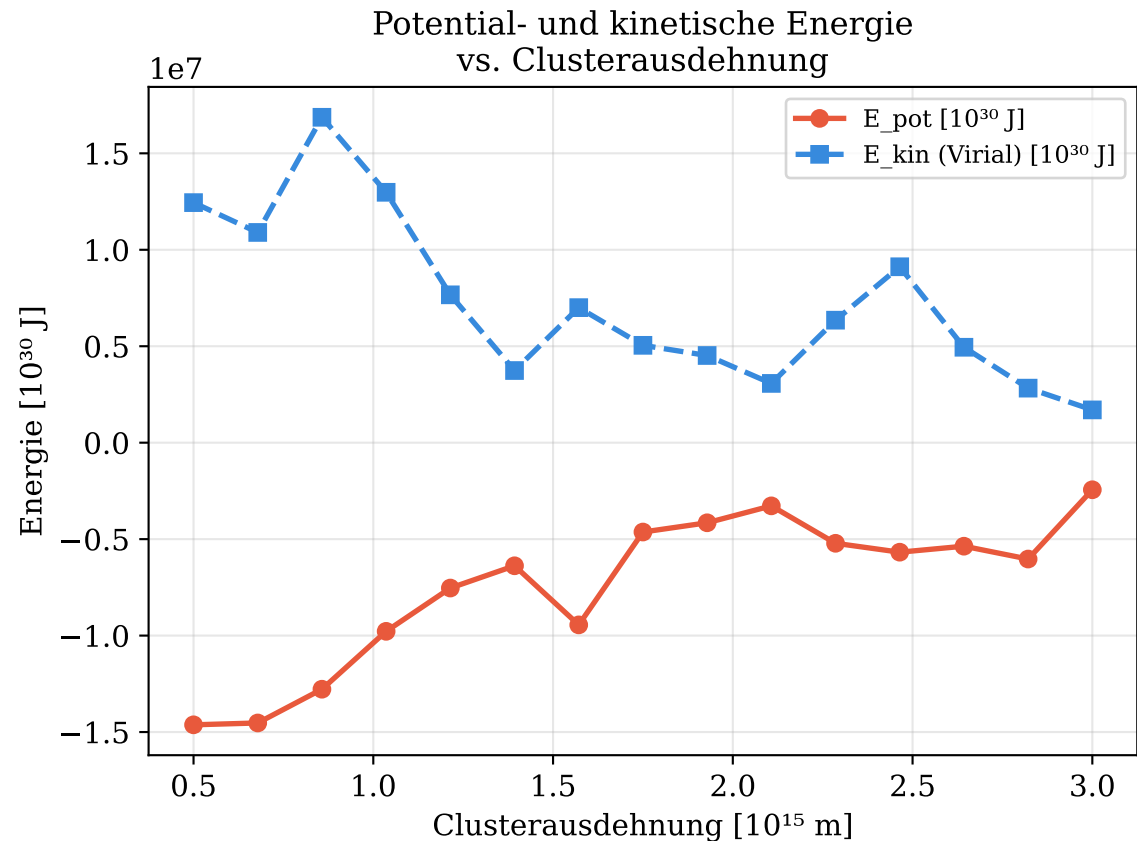
Abbildung 7: Energetik der Sterncluster — Virial-Theorem-Analyse
