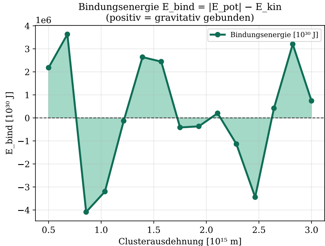
Abbildung 7: Energetik der Sterncluster — Virial-Theorem-Analyse
