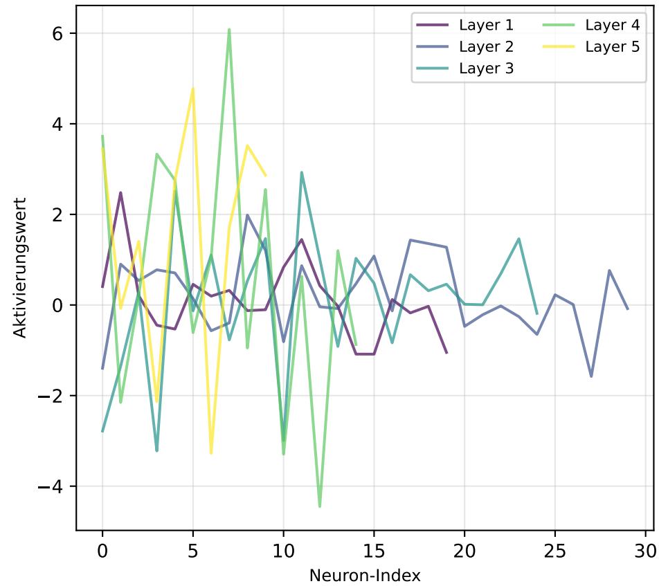
Forward-Propagation (Aktivierungen)
