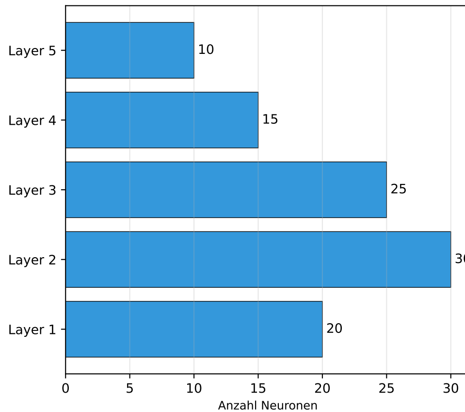
Netzwerk-Architektur
