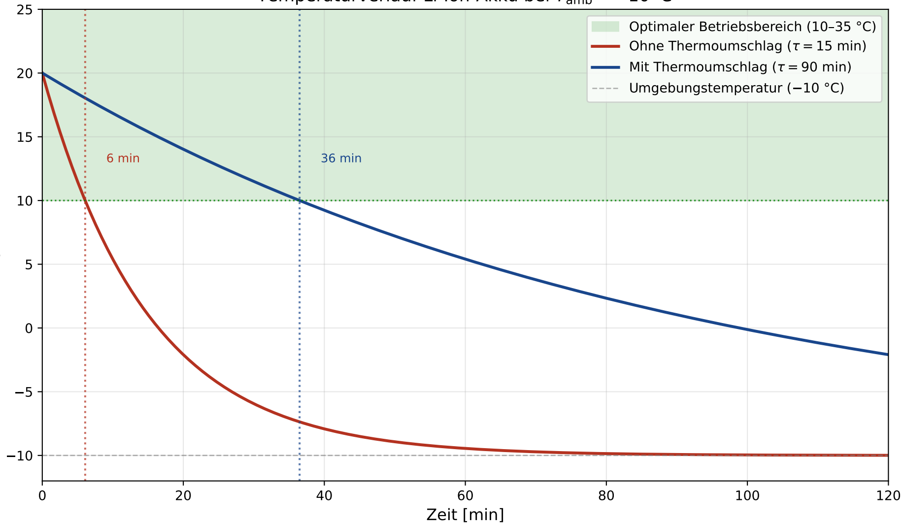
Temperaturverlauf Li-Ion-Akku bei T_{\text{amb}} = -10\text{ °C}
