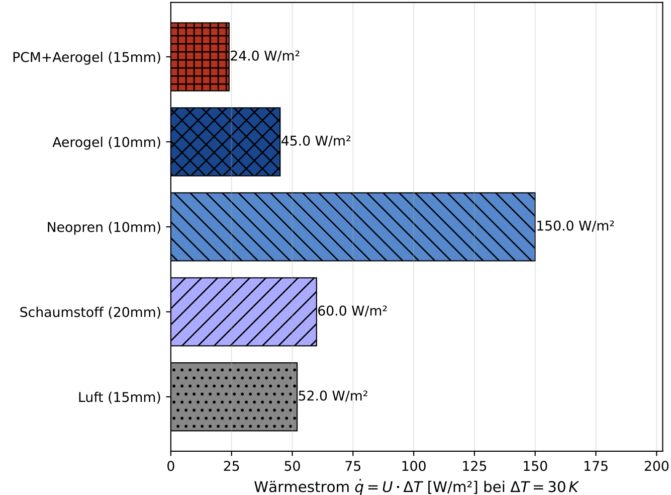
Wärmeverlust durch die Dämmschicht
