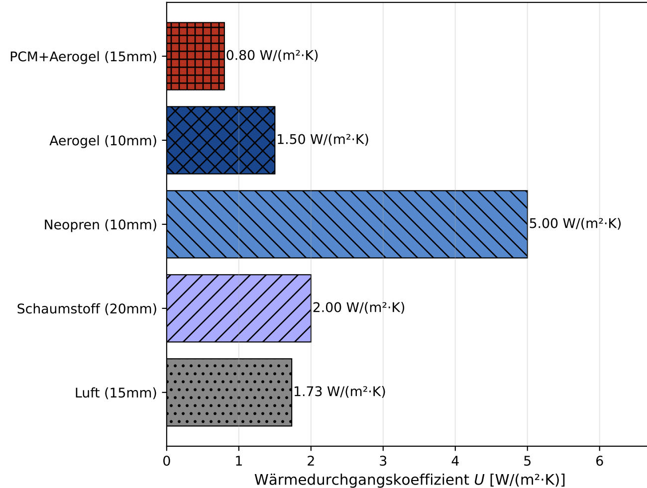
U-Werte verschiedener Isolationsmaterialien
