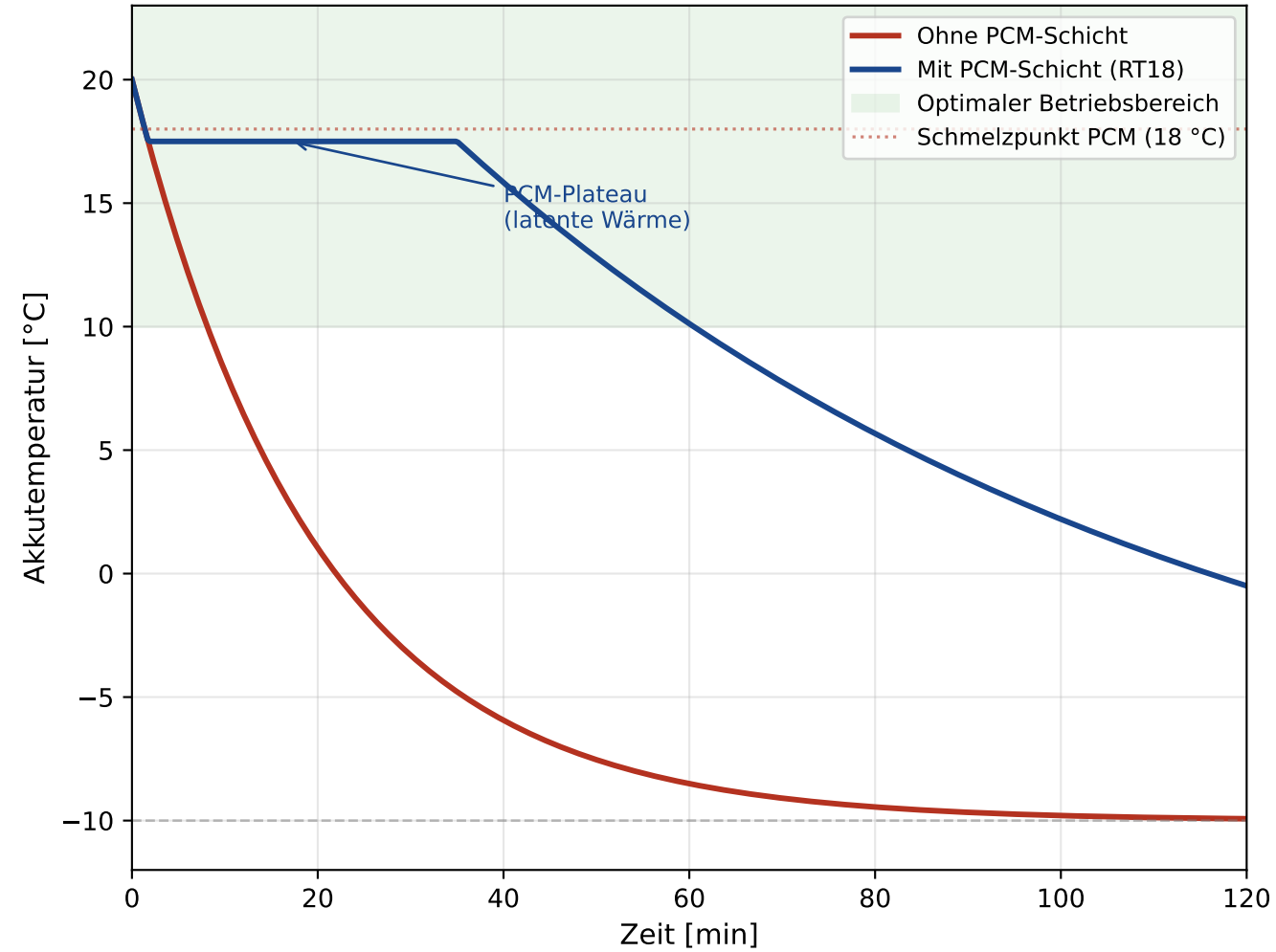
PCM-Pufferwirkung im Zeitverlauf
