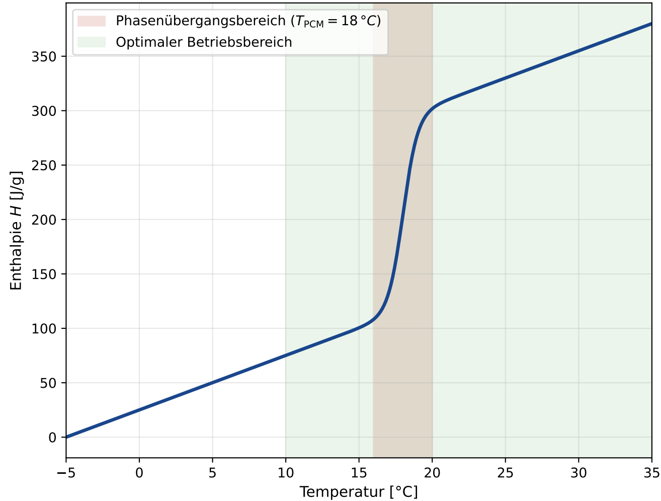
Enthalpie-Kurve PCM (RT18-Paraffin)
