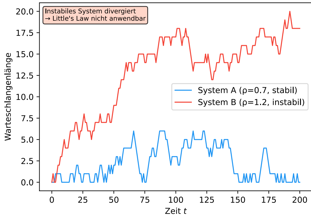
Warteschlangenlänge: A (stabil) vs. B (instabil)
