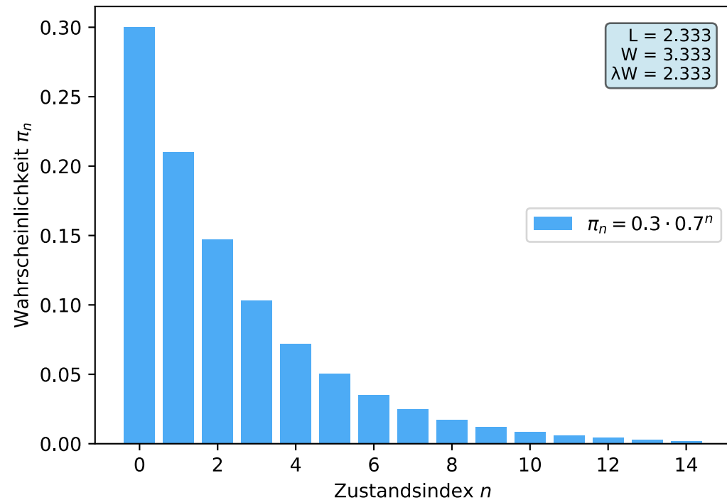
System A ( \rho=0.7 ): Stationäre Verteilung
