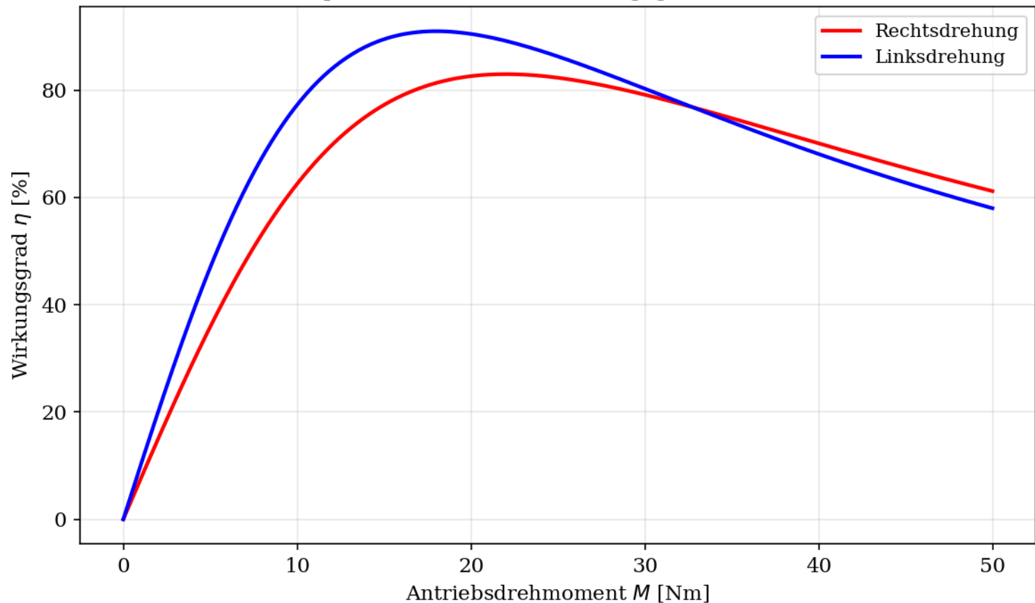
Exp. 3 - Drehmoment-Wirkungsgrad-Kennlinie
