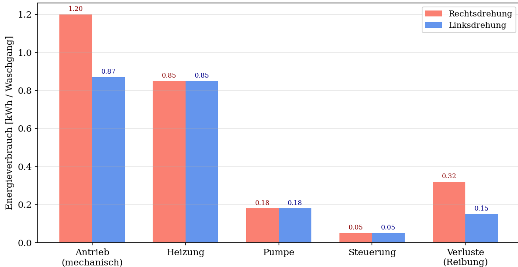
Exp. 5 - Energiebilanz eines Waschgangs (60 °C, 7 kg)
