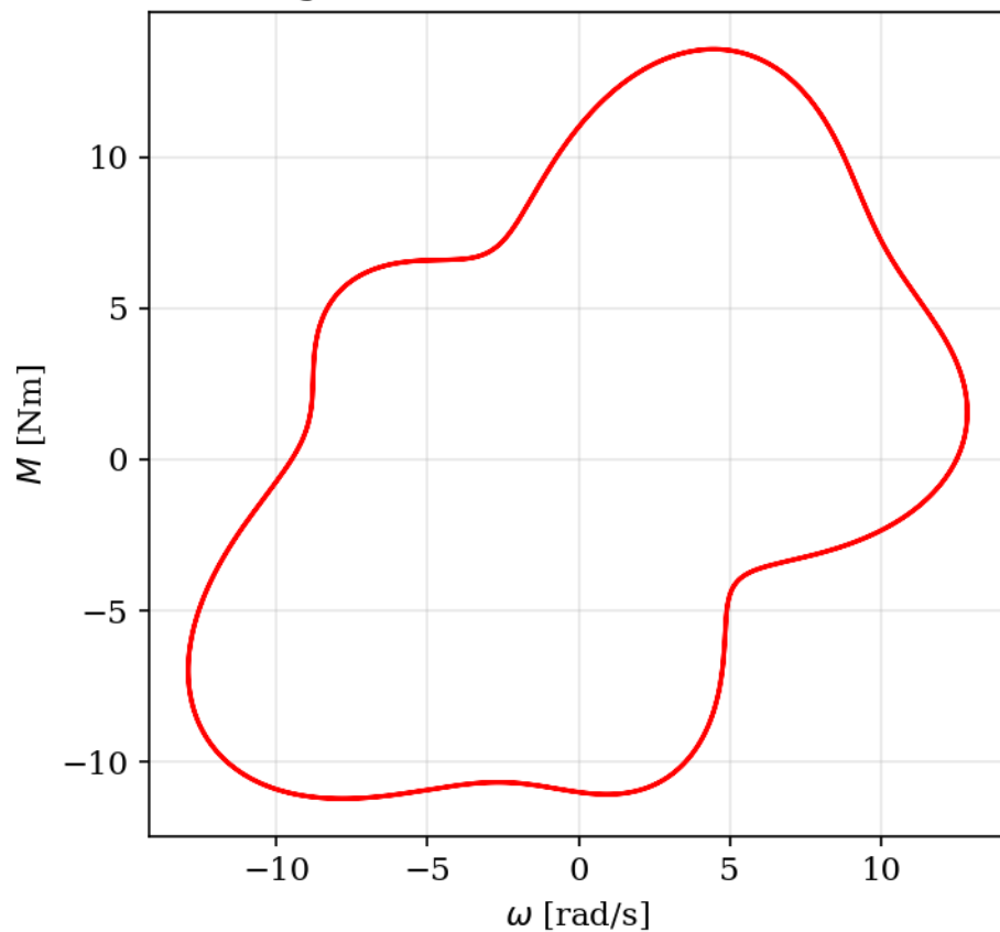
Phasenraum: Rechtsdrehung (größerer, instabilerer Attraktor)
