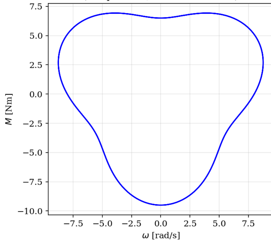
Phasenraum: Linksdrehung (kompakterer, stabilerer Attraktor)
