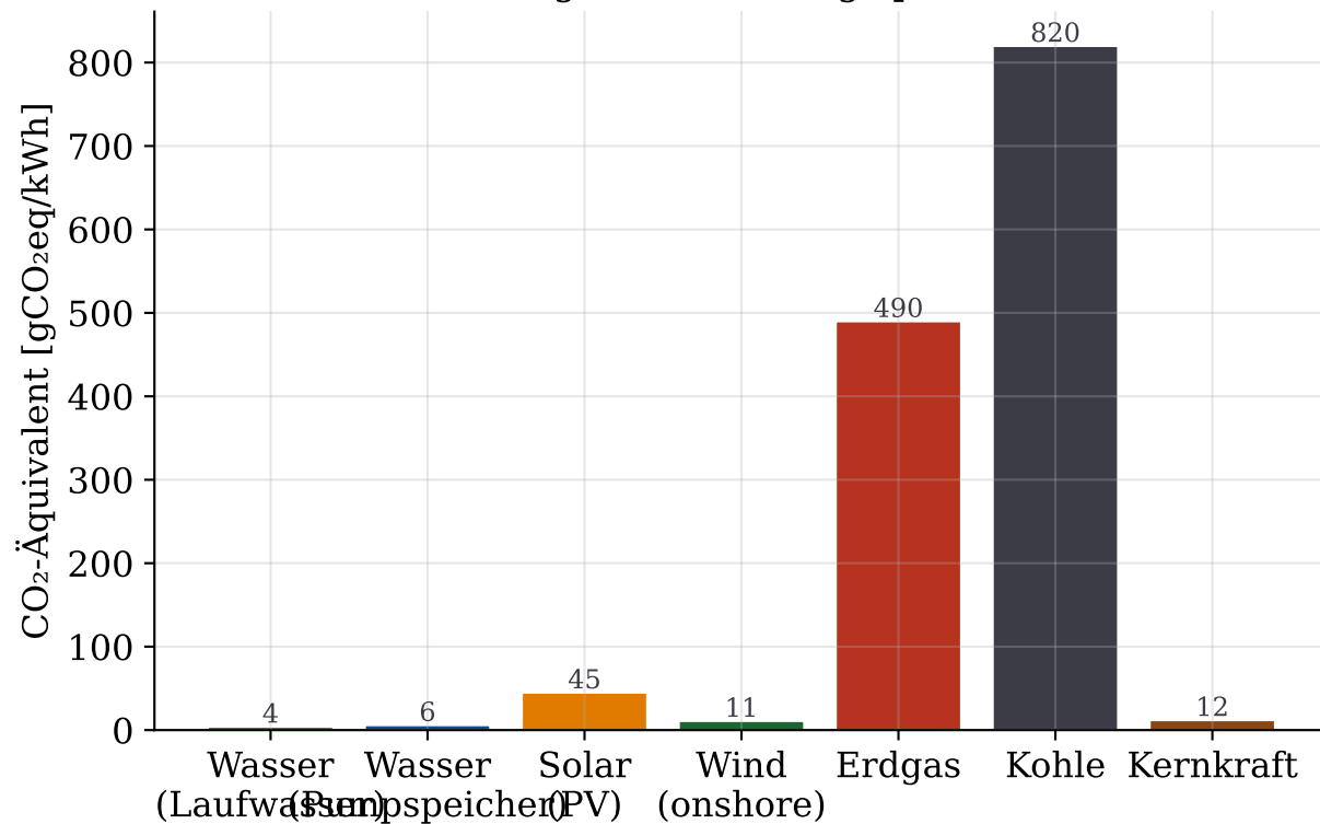
CO 2 -Emissionen verschiedener Energieumwandlungsquellen
