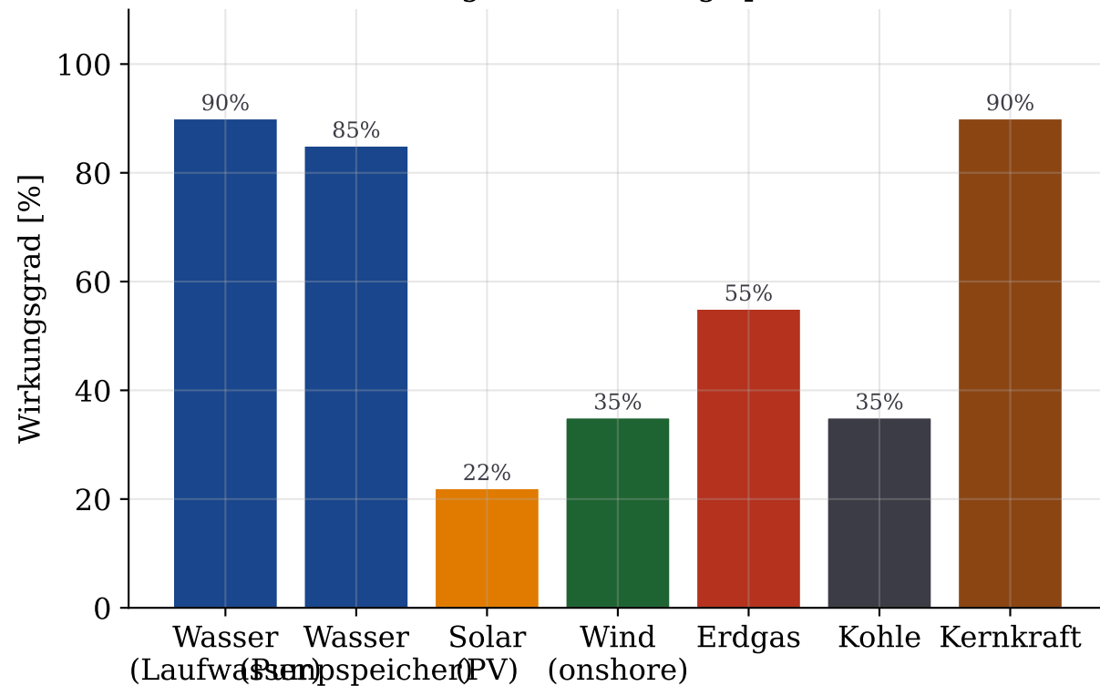
Wirkungsgrad verschiedener Energieumwandlungsquellen
