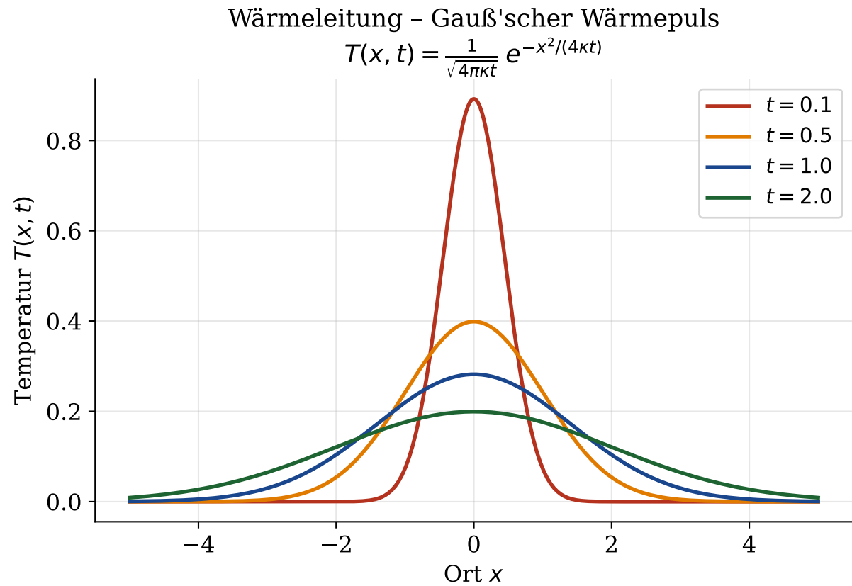
Abbildung 6: Wasser und Feuer – Temperaturkurven und Wärmeleitung
