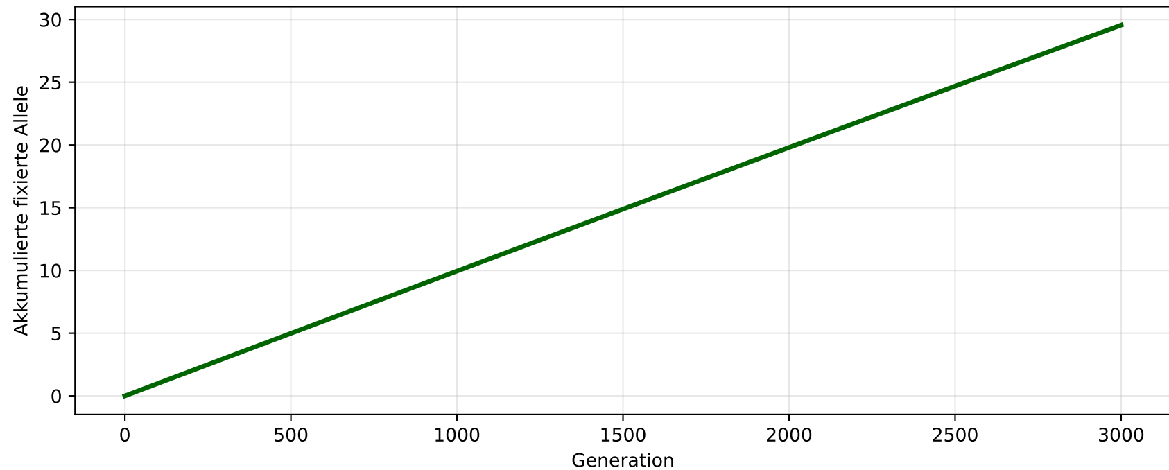
Abbildung 4: Fixierung vorteilhafter Allele nach Wright-Fisher-Modell
