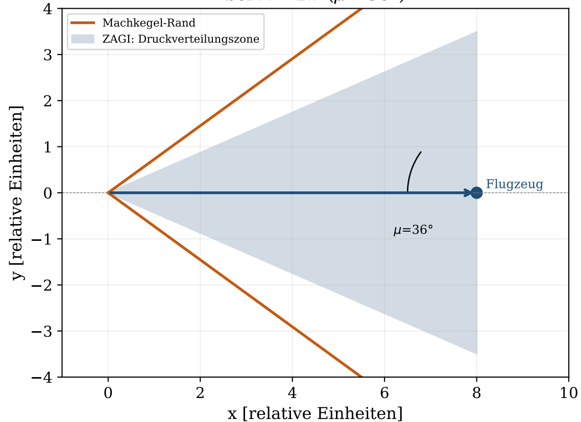
Machkegel - Schematische Darstellung bei M = 1.7 ( \mu \approx 36^\circ )
