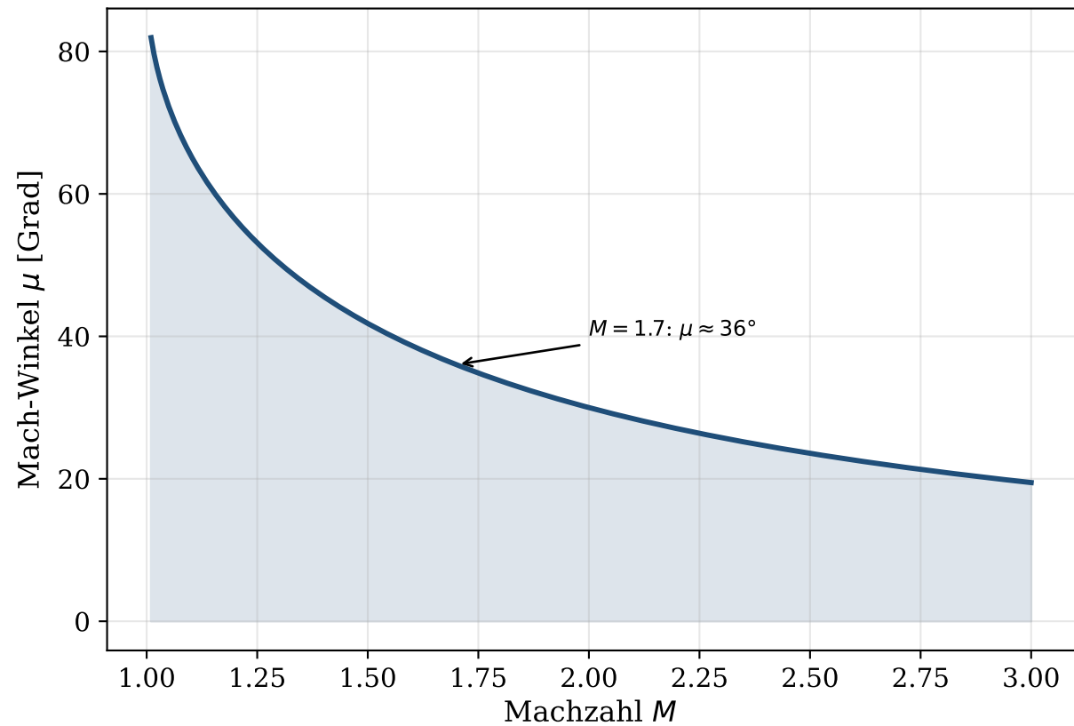
Mach-Winkel \mu = \arcsin(1/M) vs. Machzahl
